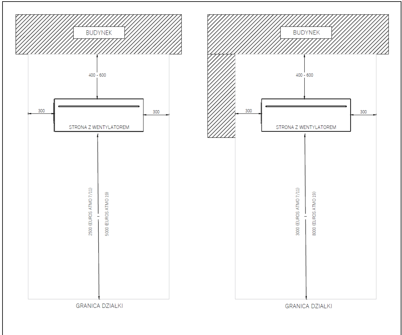
Rys. 14: Ograniczenia dotyczące miejsca ustawienia jednostki zewnętrznej pompy ciepła EUROS ATMO (wymiary w mm).
