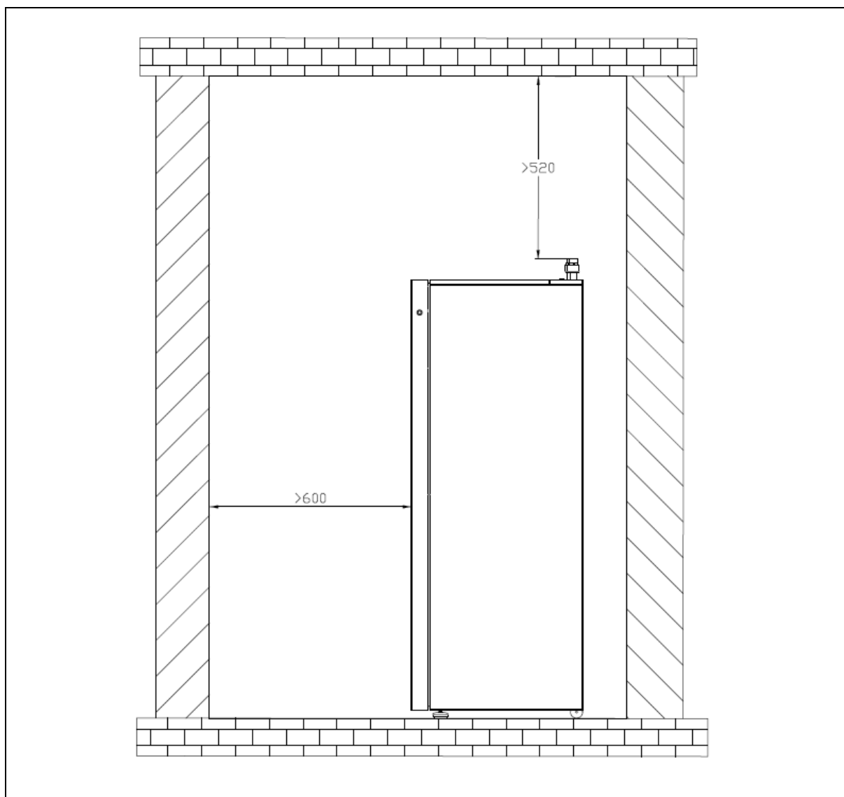
Rys. 13: Ograniczenia dotyczące miejsca ustawienia jednostki wewnętrznej pompy ciepła EUROS HYDRO 200 AIO (wymiar w mm).
