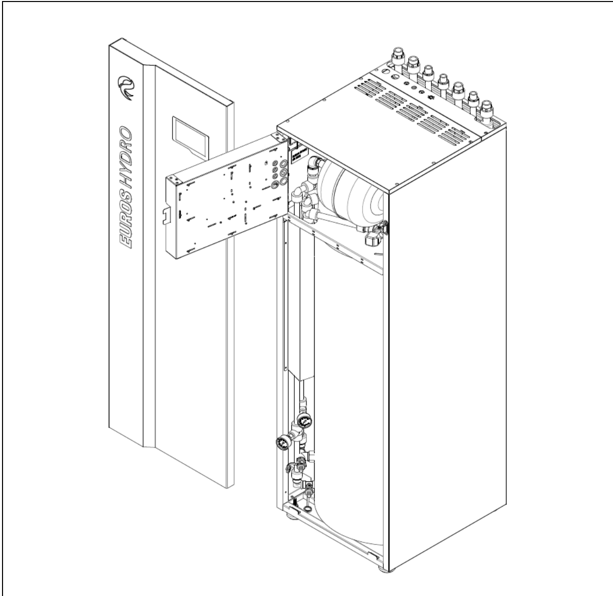
Rys. 29: Dostęp do układu hydrauliki jednostki wewnętrznej pompy ciepła EUROS HYDRO 200 AIO.
