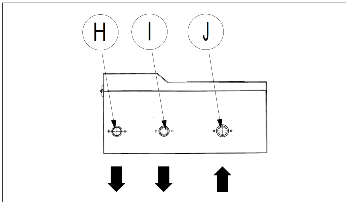
Rys. 16: Przyłącza hydrauliczne jednostki wewnętrznej pompy ciepła EUROS HYDRO 200 AIO.
