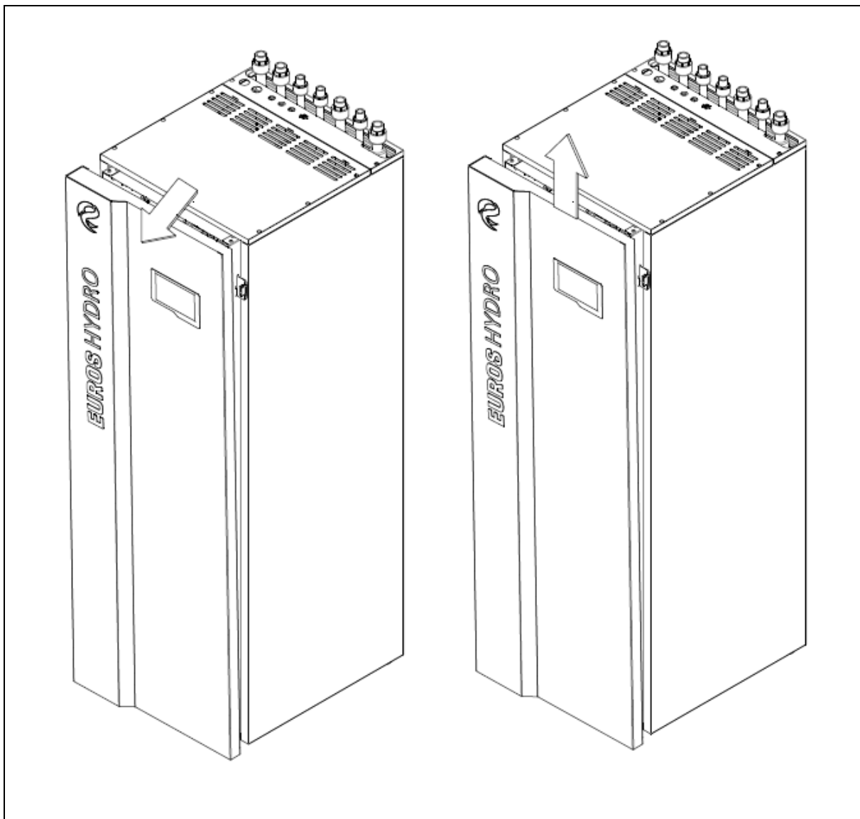
Rys. 22: Sposób otwierania frontowej osłony jednostki wewnętrznej pompy ciepła EURO HYDRO 200 AIO.
