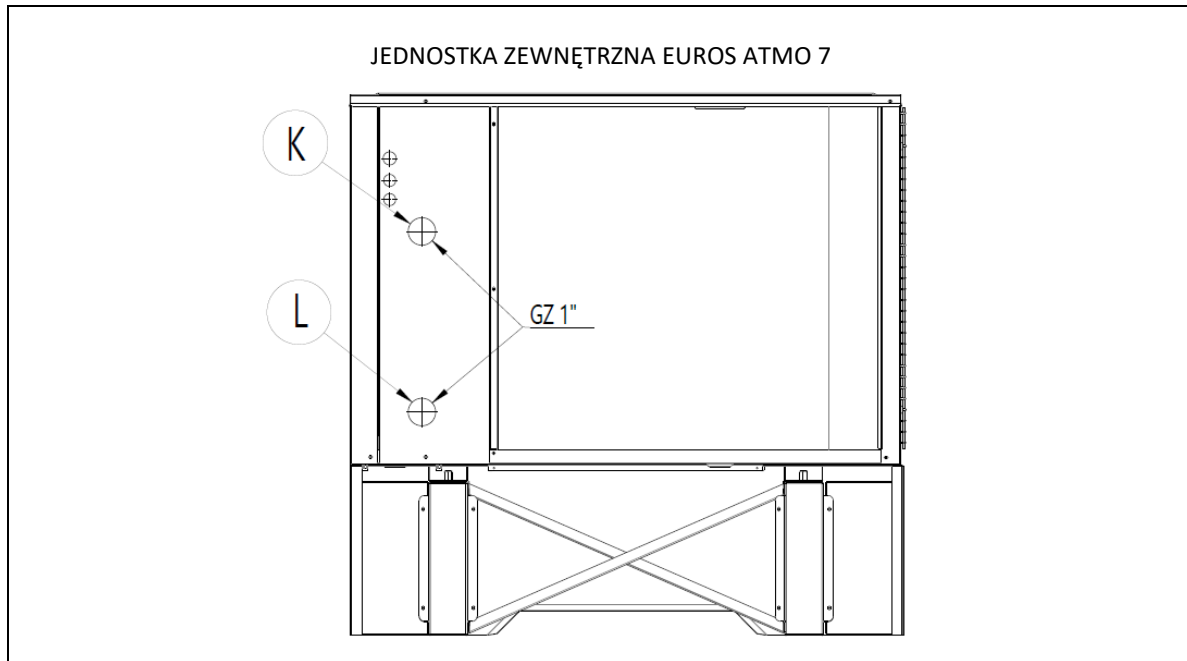
Rys. 17: Przyłącza hydrauliczne jednostki zewnętrznej pompy ciepła EUROS ATMO 7.
