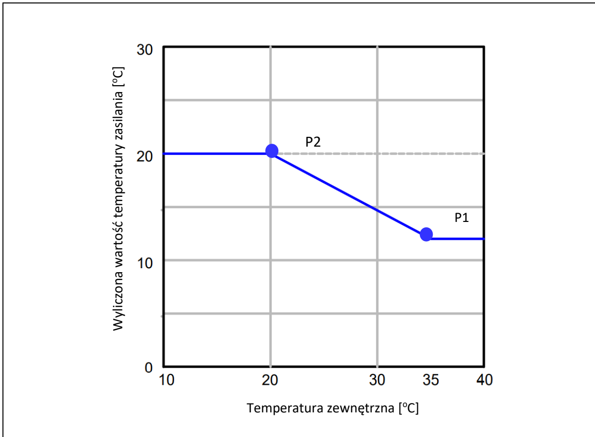
Rys. 24: Wykres krzywej chłodzenia.
