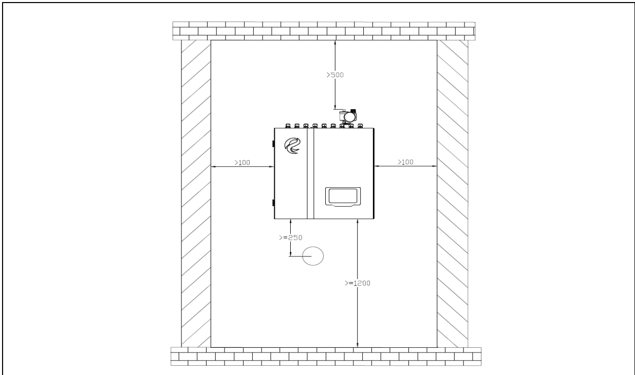
Rys. 12: Ograniczenia dotyczące miejsca ustawienia jednostki wewnętrznej pompy ciepła EUROS ATMO (wymiary w mm).
