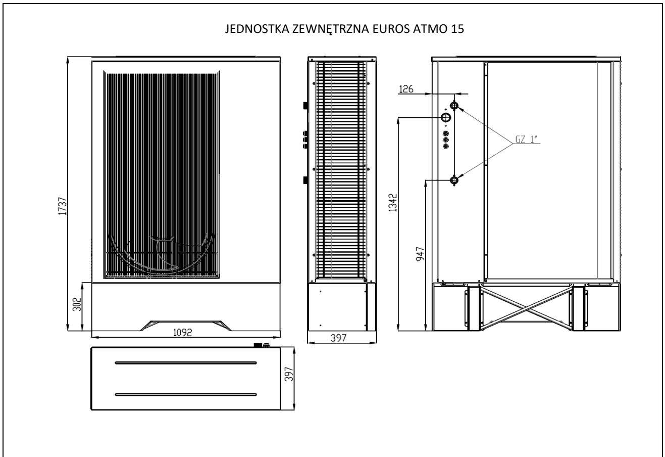
Rys. 10: Gabaryty jednostki zewnętrznej pompy ciepła EUROS ATMO 15
