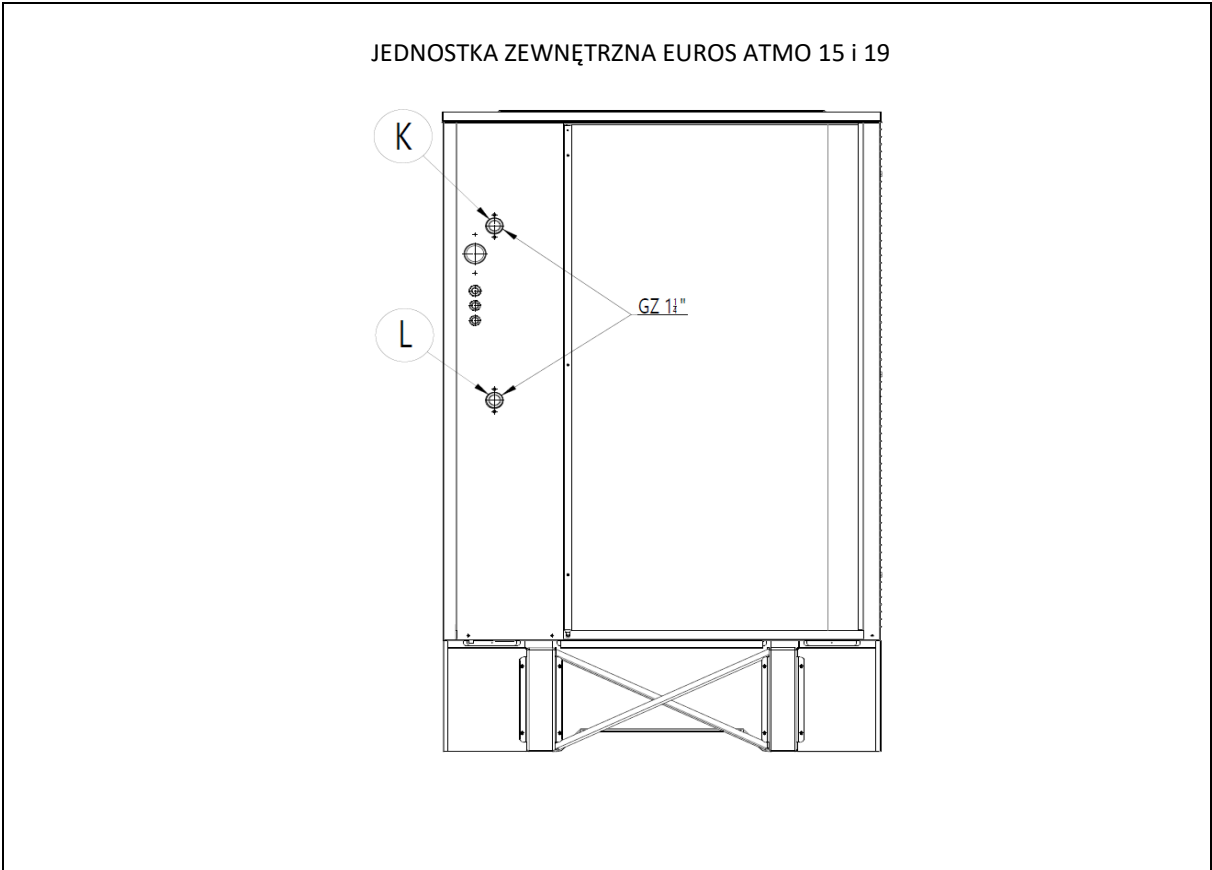
Rys. 19: Przyłącza hydrauliczne jednostki zewnętrznej pompy ciepła EUROS ATMO 15 i 19.
