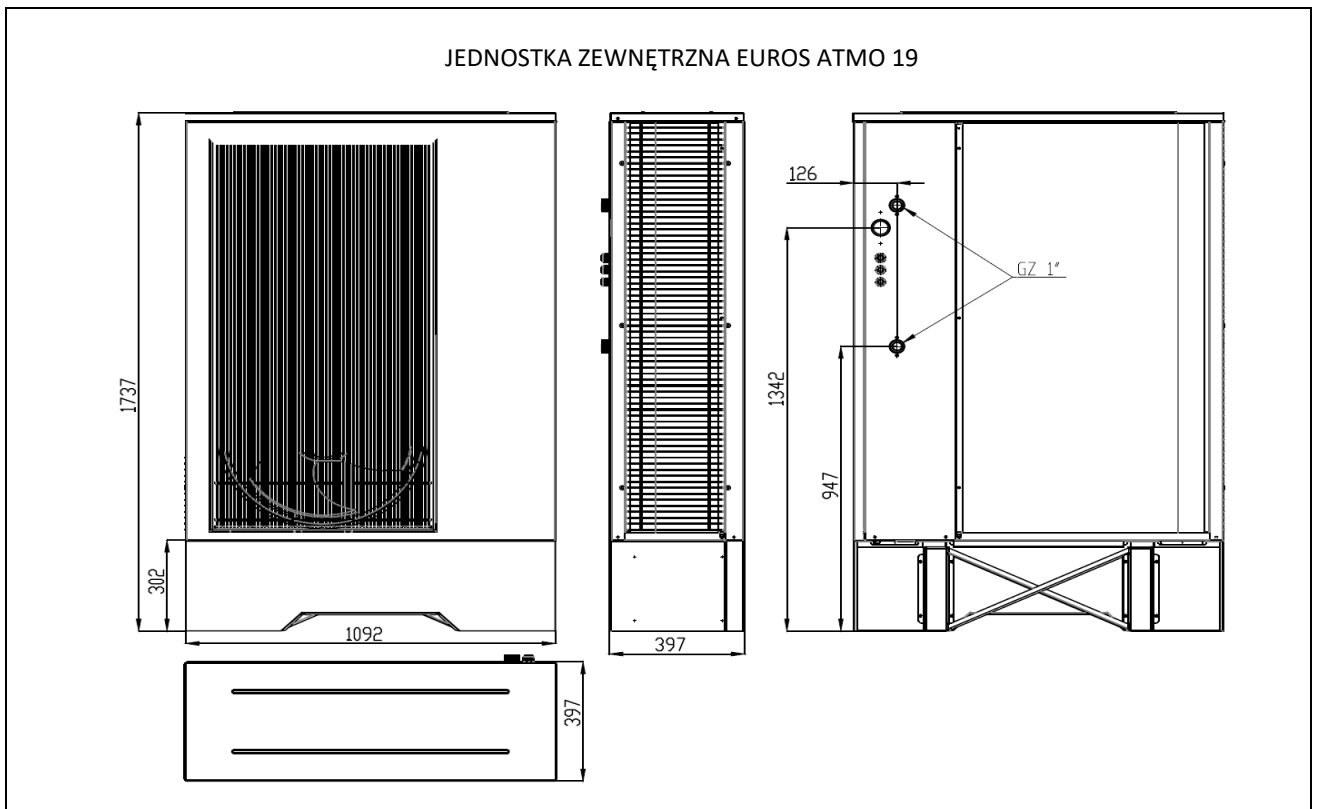
Rys. 11: Gabaryty jednostki zewnętrznej pompy ciepła EUROS ATMO 19
