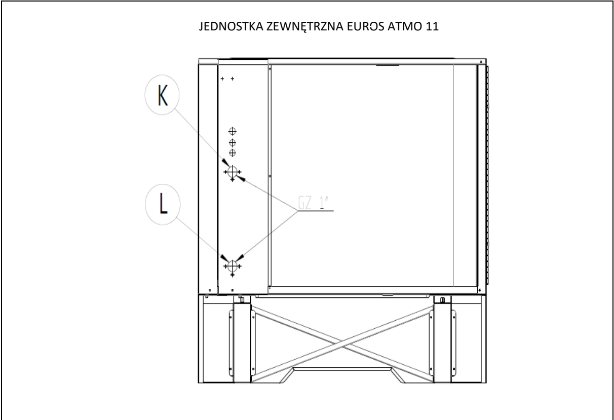
Rys. 18: Przyłącza hydrauliczne jednostki zewnętrznej pompy ciepła EUROS ATMO 11.
