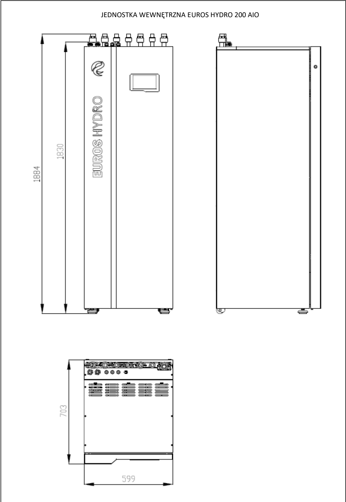
Rys. 6: Gabaryty jednostki wewnętrznej pompy ciepła EUROS HYDRO 200 AIO.
