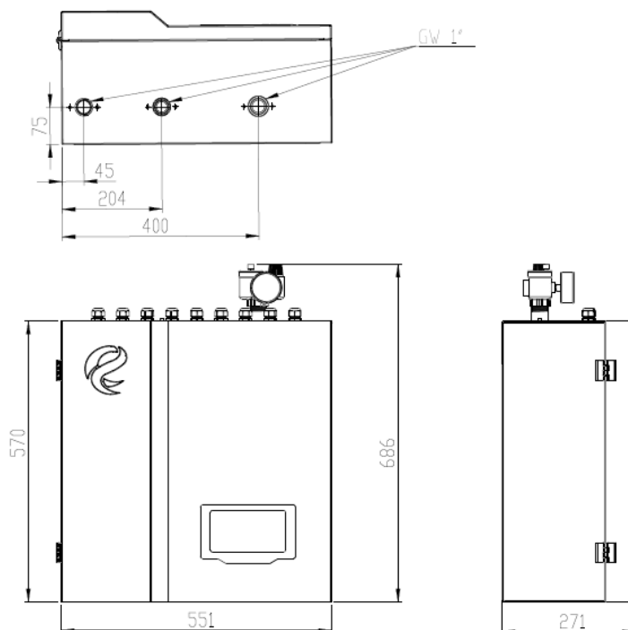
Rys. 6: Gabaryty jednostki wewnętrznej pompy ciepła EUROS ATMO
