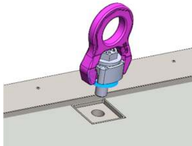
Rys. 6: Punkt mocujący w pompie ciepła EUROS CONTIBLOC MINI
