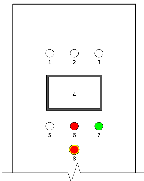
Rys.21: Widok drzwi tablicy rozdzielczej w pompie ciepła EUROS CONTIBLOC MINI
