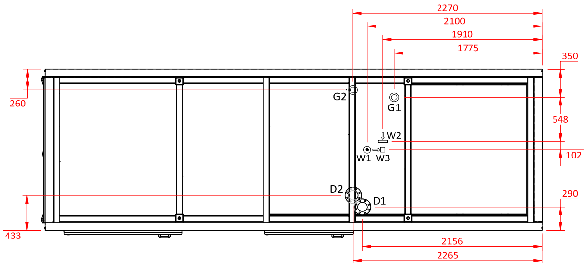
Rys. 13: Umiejscowienie przyłączy hydraulicznych w odniesieniu do podstawy pompy ciepła EUROS CONTIBLOC MINI
