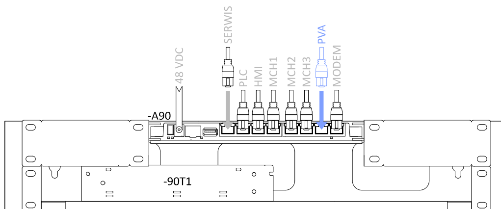
Rys. 40: Widok części komunikacyjnej głównej szafy automatyki i miejsce przyłączenia sygnałów komunikacyjnych z falowników PV dla wersji układu elektrycznego ECx12, ECx13
