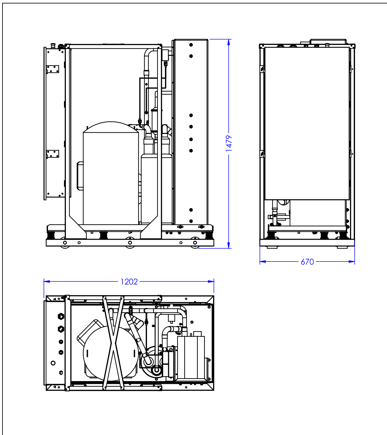
Rys. 3: Gabaryty jednostki wewnętrznej pompy ciepła EUROS GEO PRO 2.
