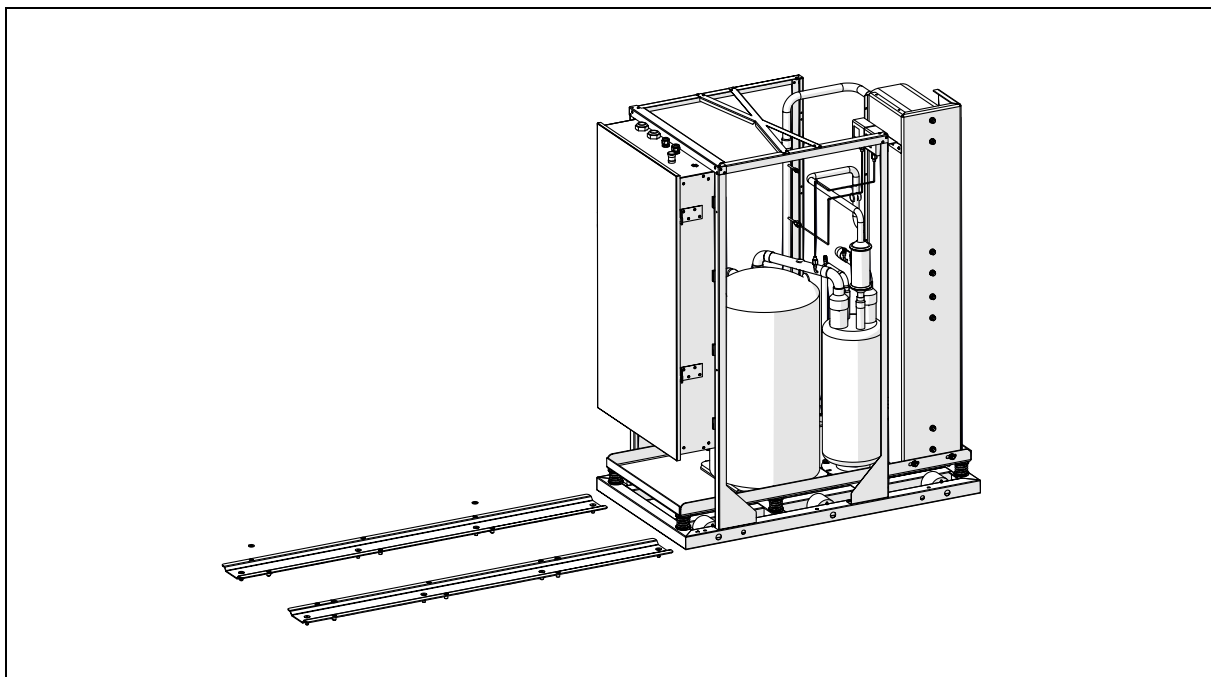
Rys. 6: Przygotowanie pompy ciepła do montażu.
