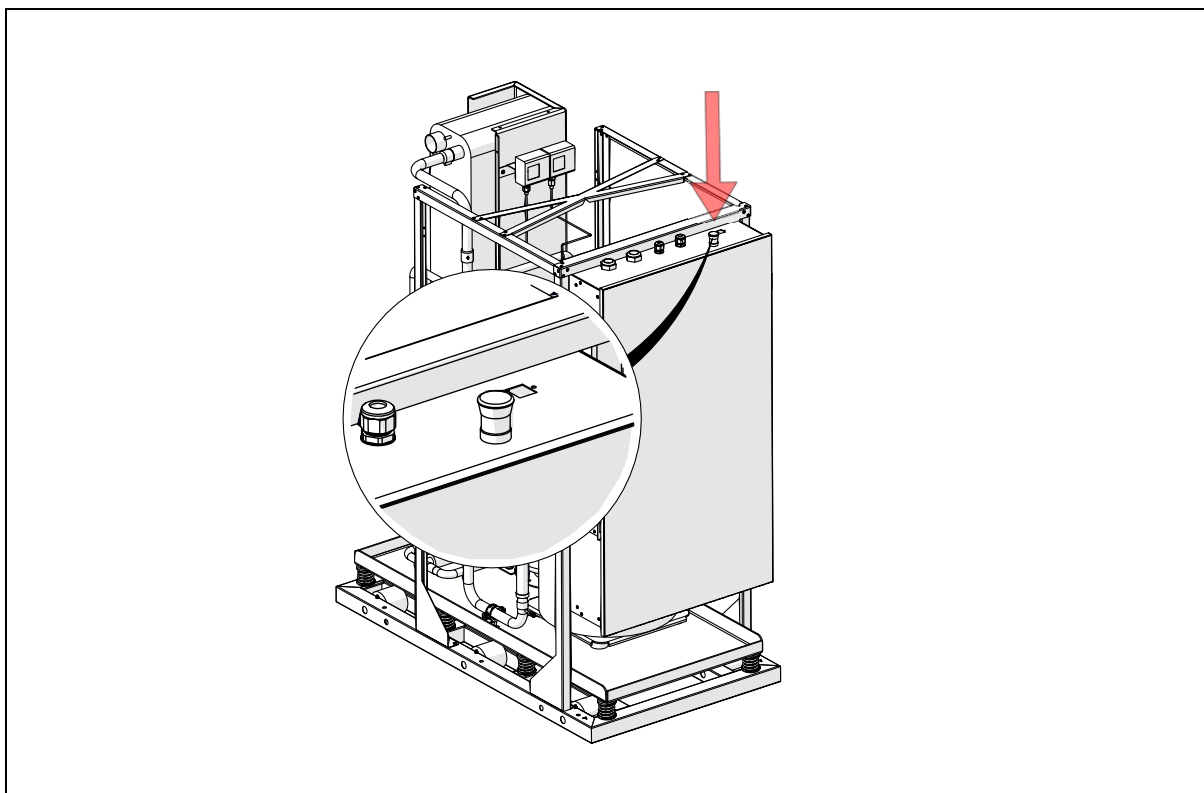
Rys. 15: Awaryjne zatrzymanie pompy ciepła przez wciśnięcie przycisku awaryjnego.
