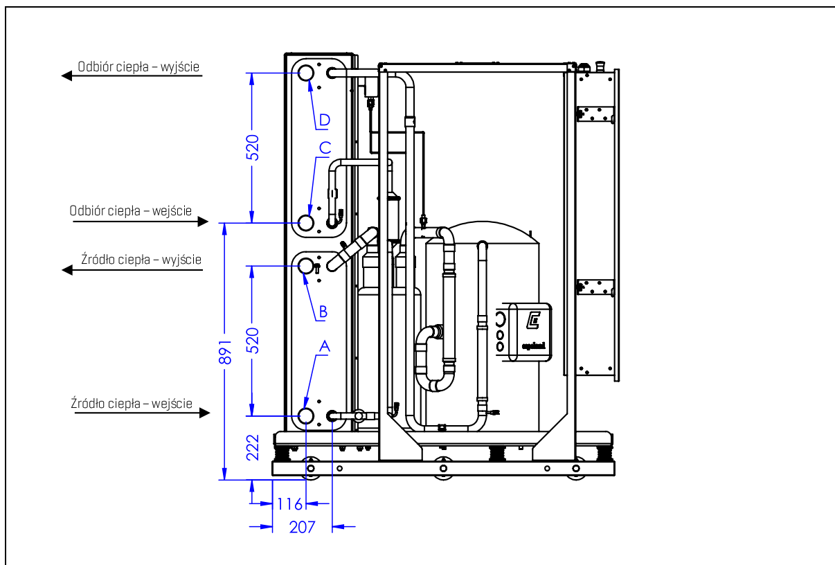
Rys. 11: Tylna strona obudowy pompy ciepła EUROS GEO PRO 2.
