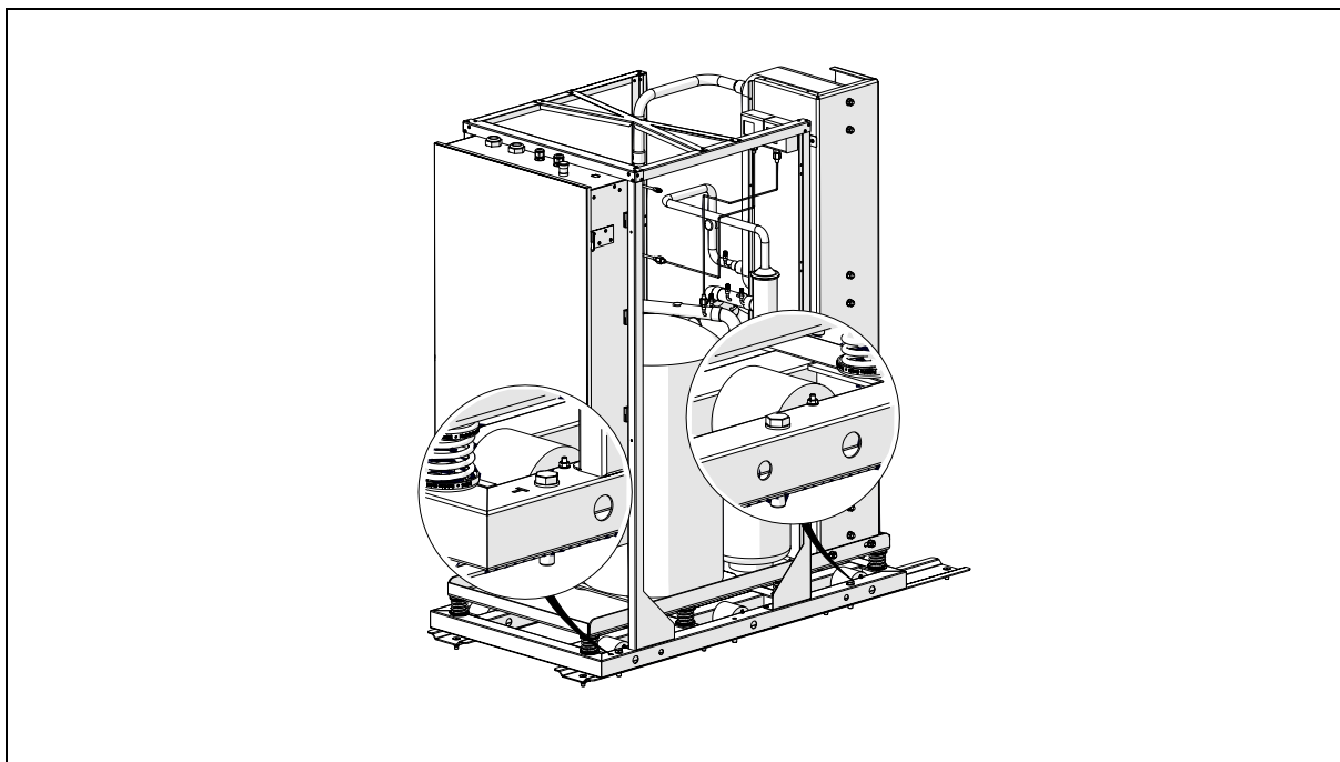
Rys. 10: Wkręcenie śrub blokujących w ramę modułu pompy ciepła.
