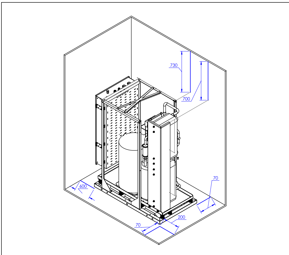
Rys. 5: Ograniczenia dotyczące miejsca ustawienia pompy ciepła EUROS GEO PRO 2 z wyjątkiem pracy w kaskadzie.
