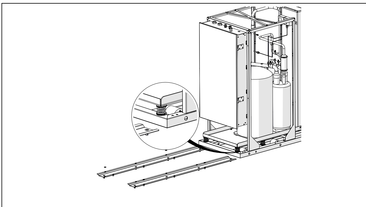
Rys. 7: Nakierowanie pompy ciepła na szyny montażowe.
