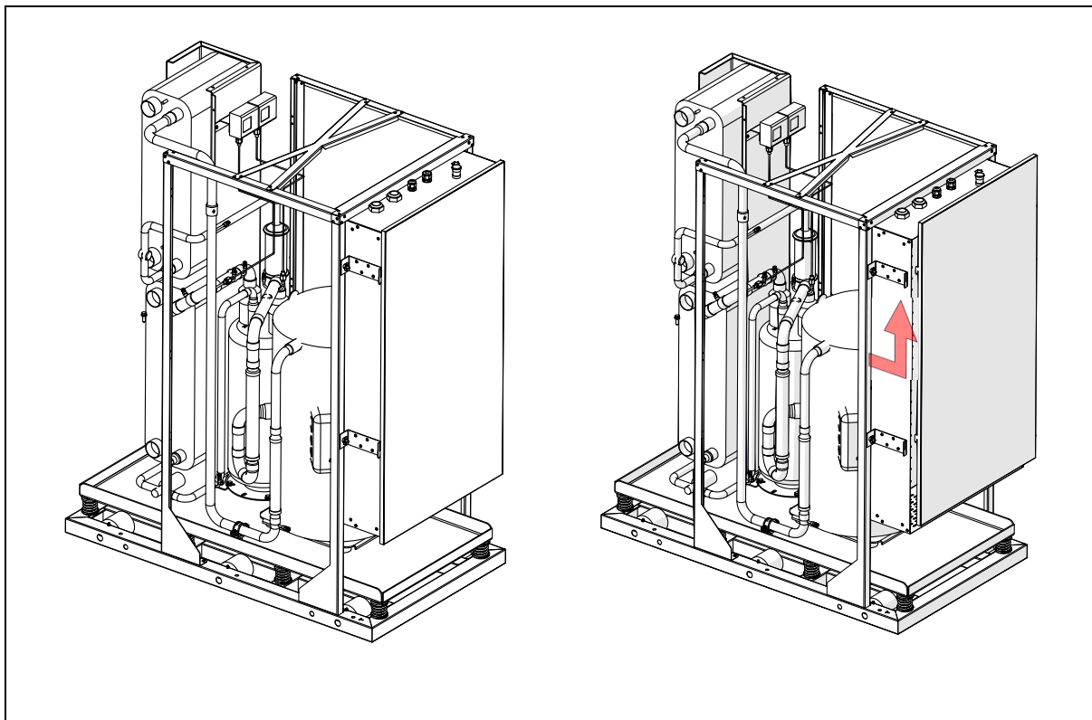
Rys. 14: Sposób zdejmowania panelu frontowego pompy ciepła EUROS GEO PRO 2.
