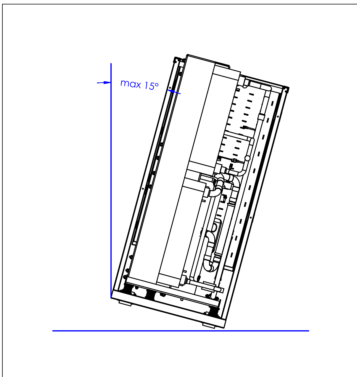
Rys. 4: Maksymalny przechył pompy ciepła EUROS GEO PRO 2 w czasie transportu.
