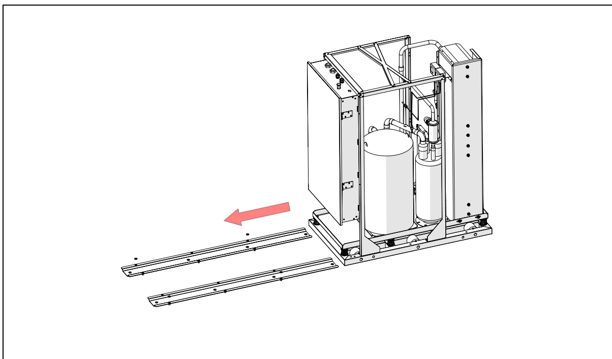
Rys. 8: Wsuniecie pompy ciepła na szyny montażowe.
