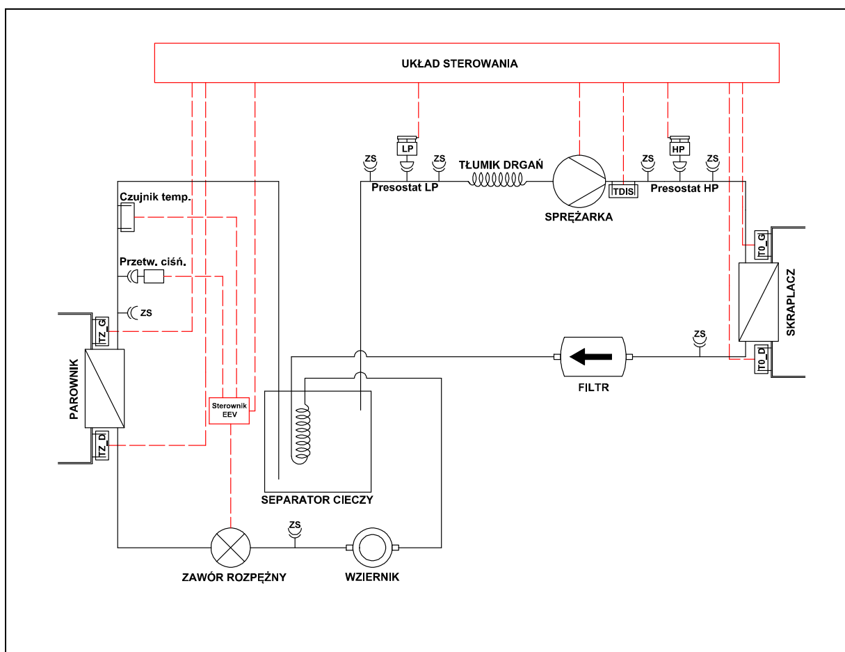
Rys. 2: Ogólny schemat układu chłodniczego i układu sterowania w pompach ciepła EUROS GEO PRO 2 54 MT/HT (ETM6-CTM3) oraz EUROS GEO PRO 2 28 MT/HT (ETM6-CTM3).
