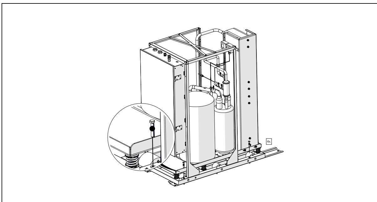
Rys.9: Wsuniecie śrub blokujących w otwory umieszczone w ramie.
