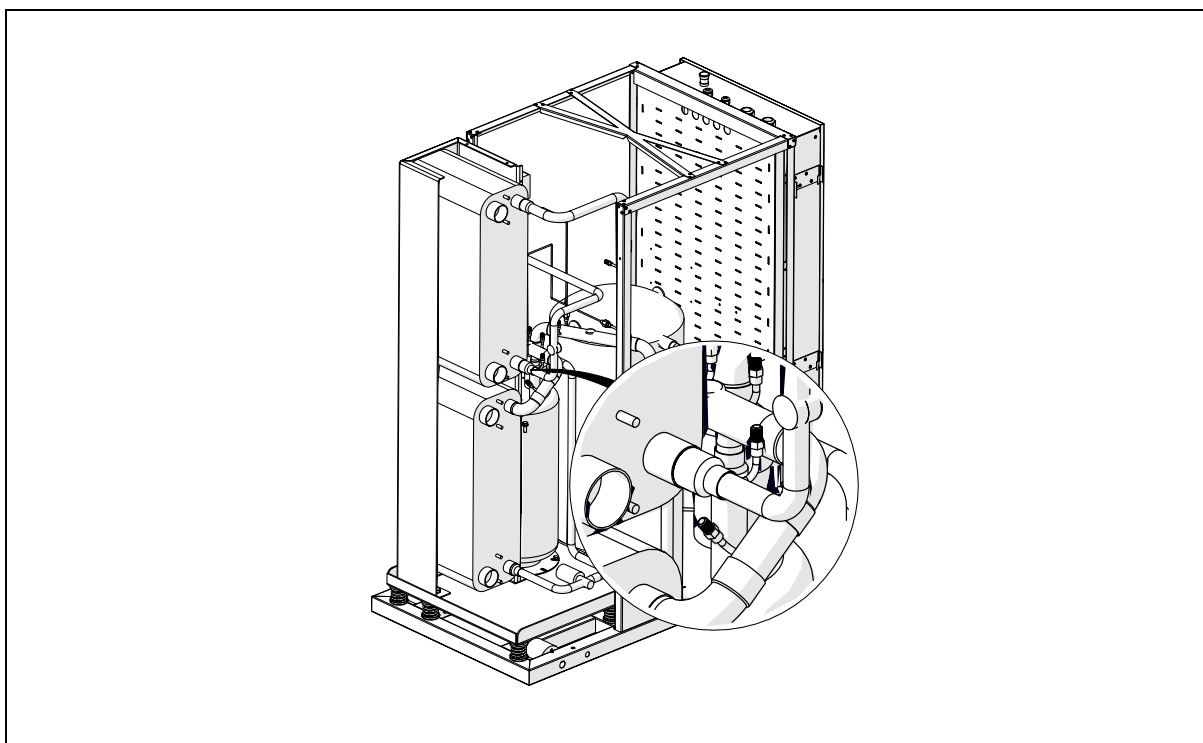
Rys. 16: Usytuowanie zaworów serwisowych w pompie ciepła EUROS GEO PRO 2.
