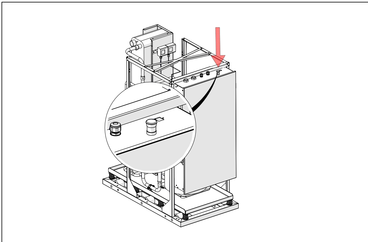
Rys. 51: Awaryjne zatrzymanie pompy ciepła przez wciśnięcie przycisku awaryjnego.
