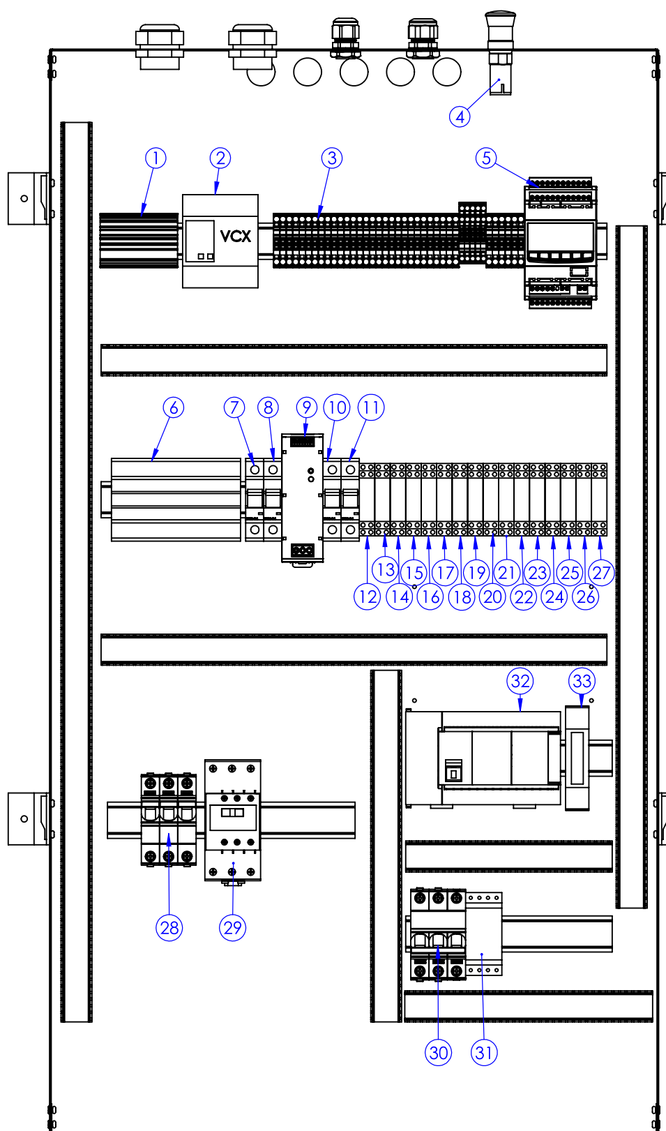
Rys. 46: Tablica elektryczna pompy ciepła EUROS GEO PRO 2 w wersji ETM1.
