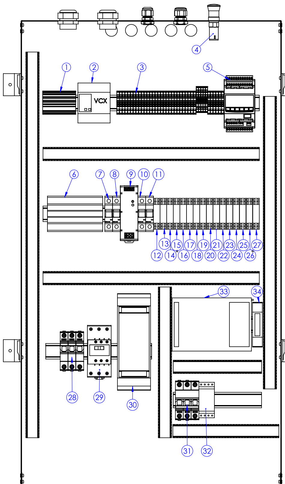
Rys. 47: Tablica elektryczna pompy ciepła EUROS GEO PRO 2 w wersji ETM2.
