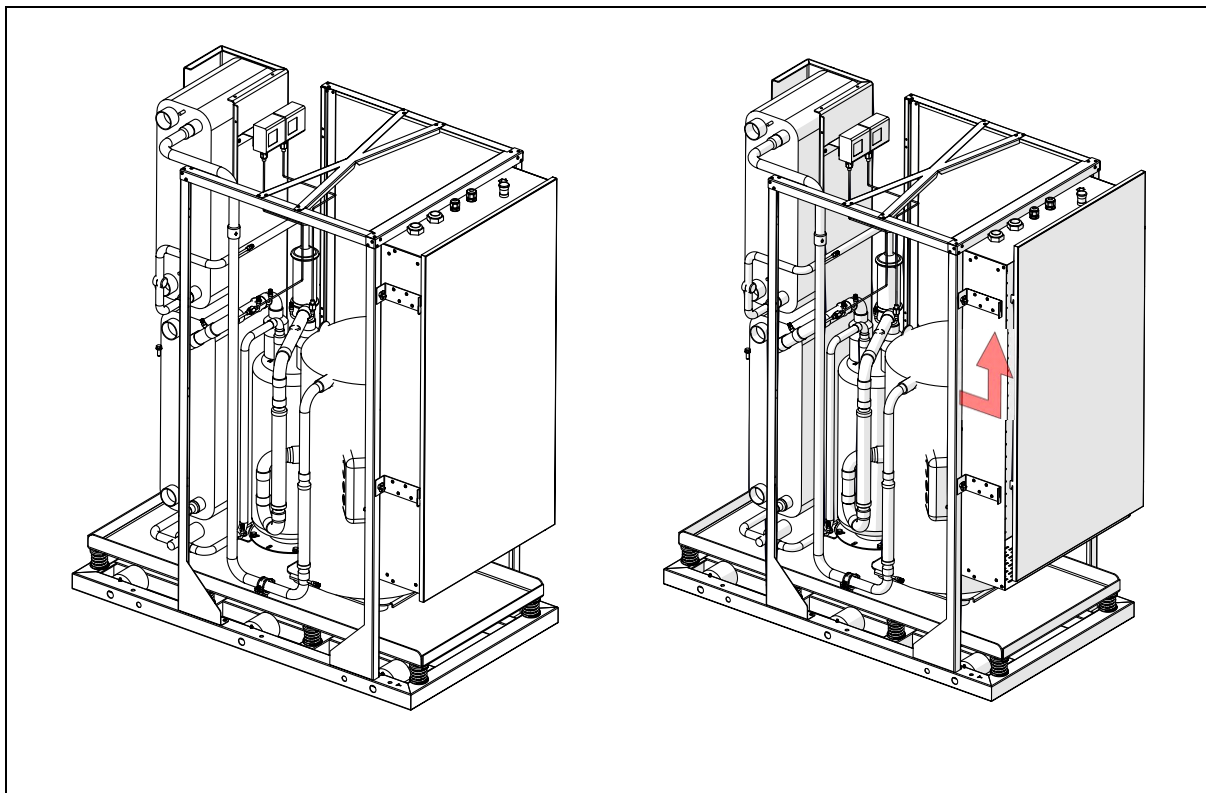
Rys. 50: Sposób zdejmowania panelu frontowego pompy ciepła EUROS GEO PRO 2.
