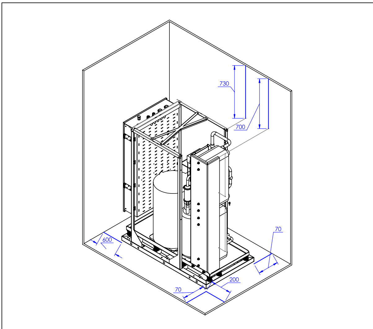
Rys. 6: Ograniczenia dotyczące miejsca ustawienia pompy ciepła EUROS GEO PRO 2 z wyjątkiem pracy w kaskadzie.
