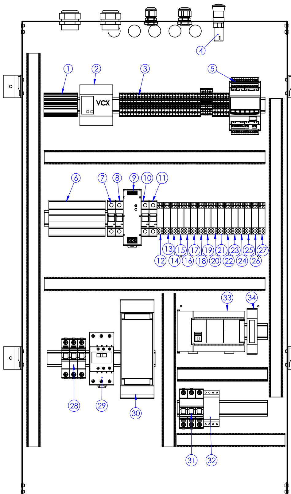
Rys. 48: Tablica elektryczna pompy ciepła EUROS GEO PRO 2 w wersji ETM3.
