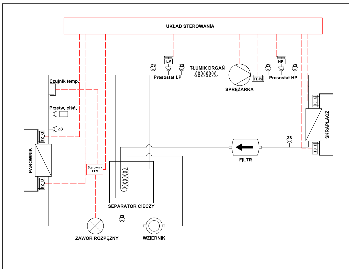
Rys. 2: Ogólny schemat układu chłodniczego i układu sterowania w pompach ciepła EUROS GEO PRO 2 54 MT/HT (ETM5-CTM3) oraz EUROS GEO PRO 2 28 MT/HT (ETM5-CTM3).
