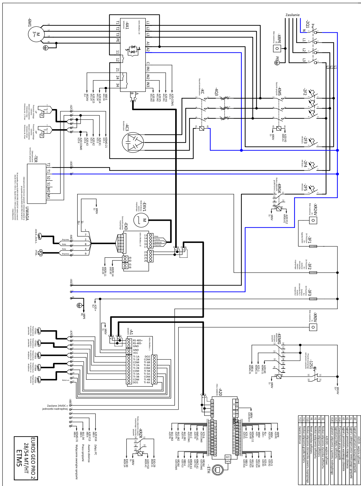
Rys. 12: Schemat elektryczny pompy ciepła EUROS GEO PRO 2
