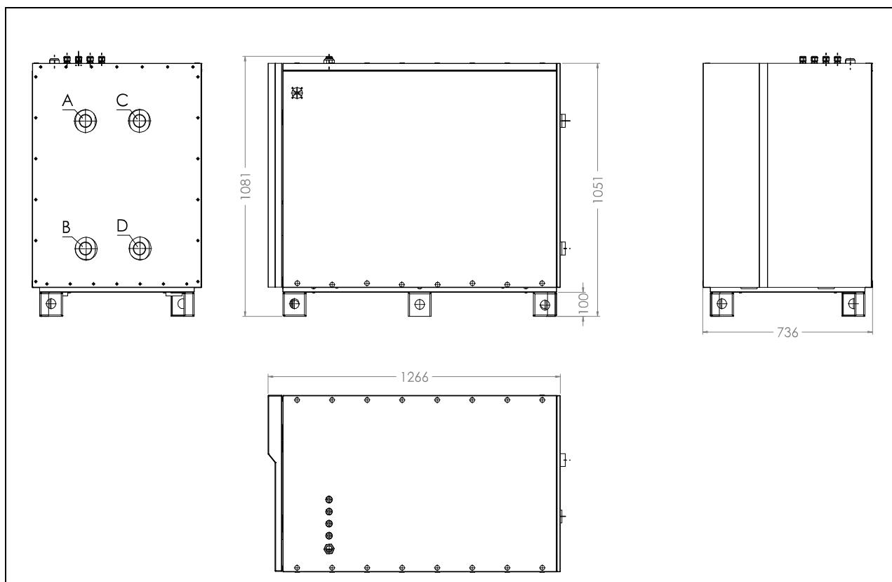
Rys. 4: Gabaryty pompy ciepła EUROS GEO PRO 3 w wersji HT.
