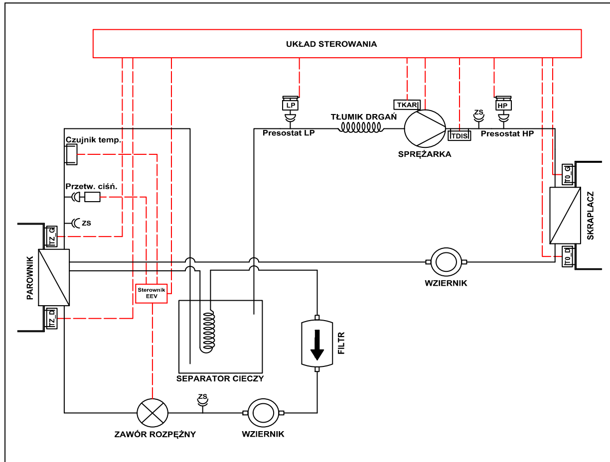
Rys. 2: Ogólny schemat układu chłodniczego i układu sterowania w pompach ciepła EUROS GEO PRO 3.
