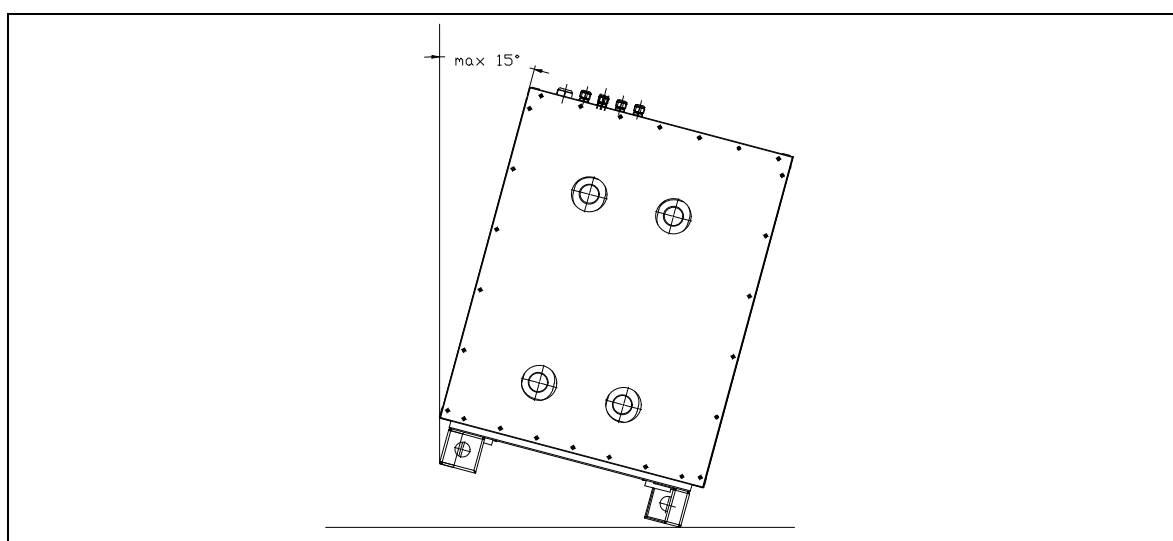
Rys. 5: Maksymalny przechył pompy ciepła EUROS GEO PRO 3 w czasie transportu.
