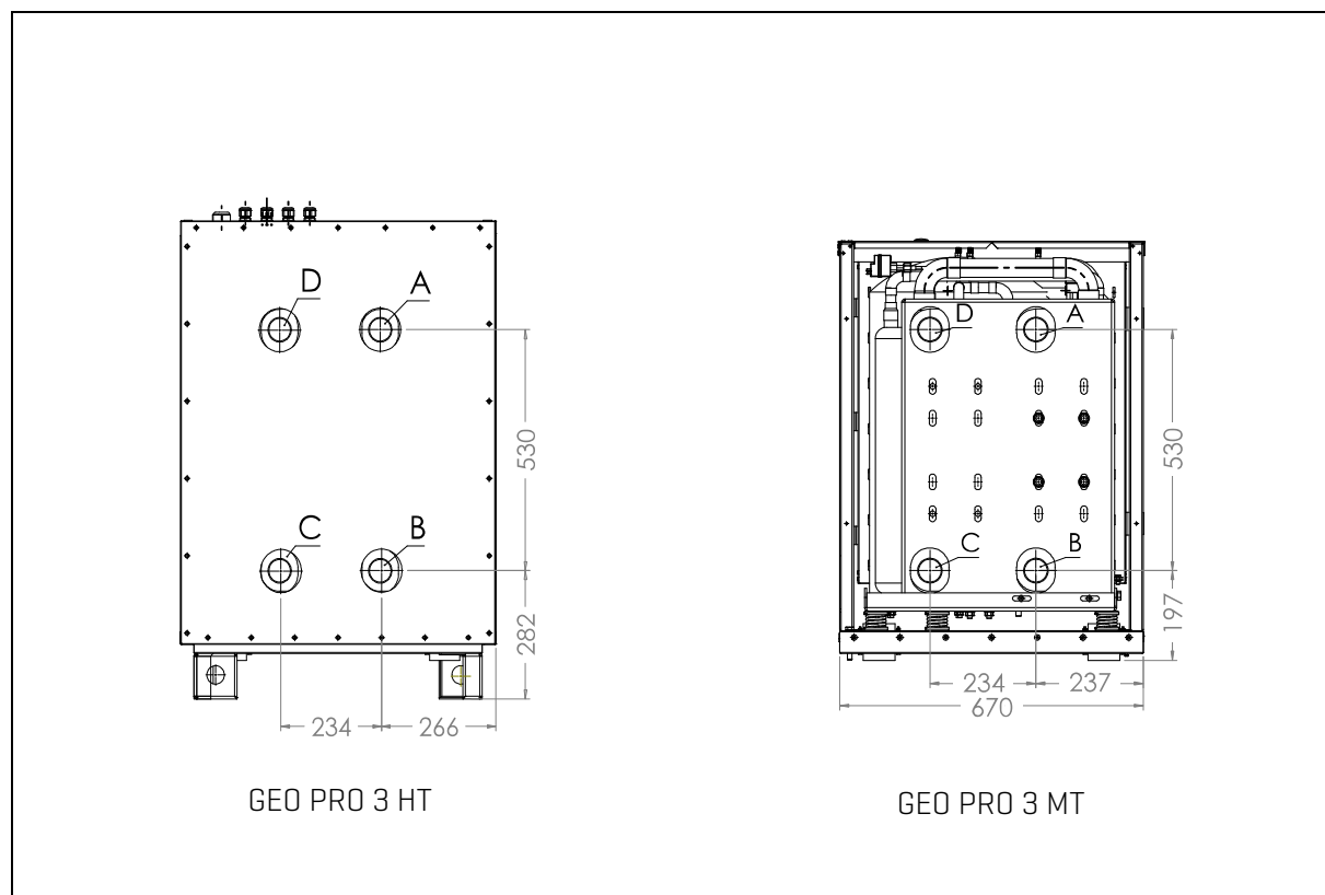
Rys. 12: Tylna strona obudowy pompy ciepła EUROS GEO PRO 3.
