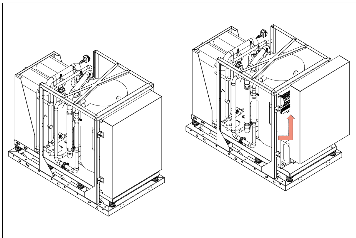
Rys. 17: Sposób zdejmowania panelu tablicy elektrycznej pompy ciepła EUROS GEO PRO 3 w wersji MT.
