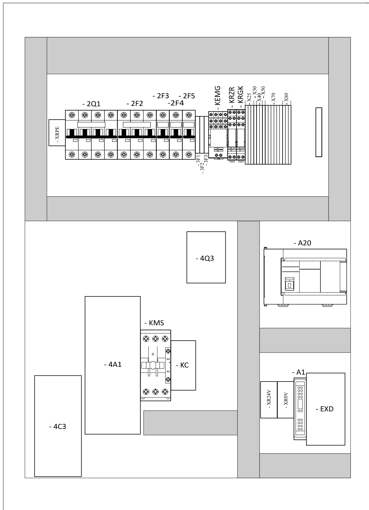
Rys. 15: Tablica elektryczna pompy ciepła EUROS GEO PRO 3 w wersji ETN1/ETN2.
