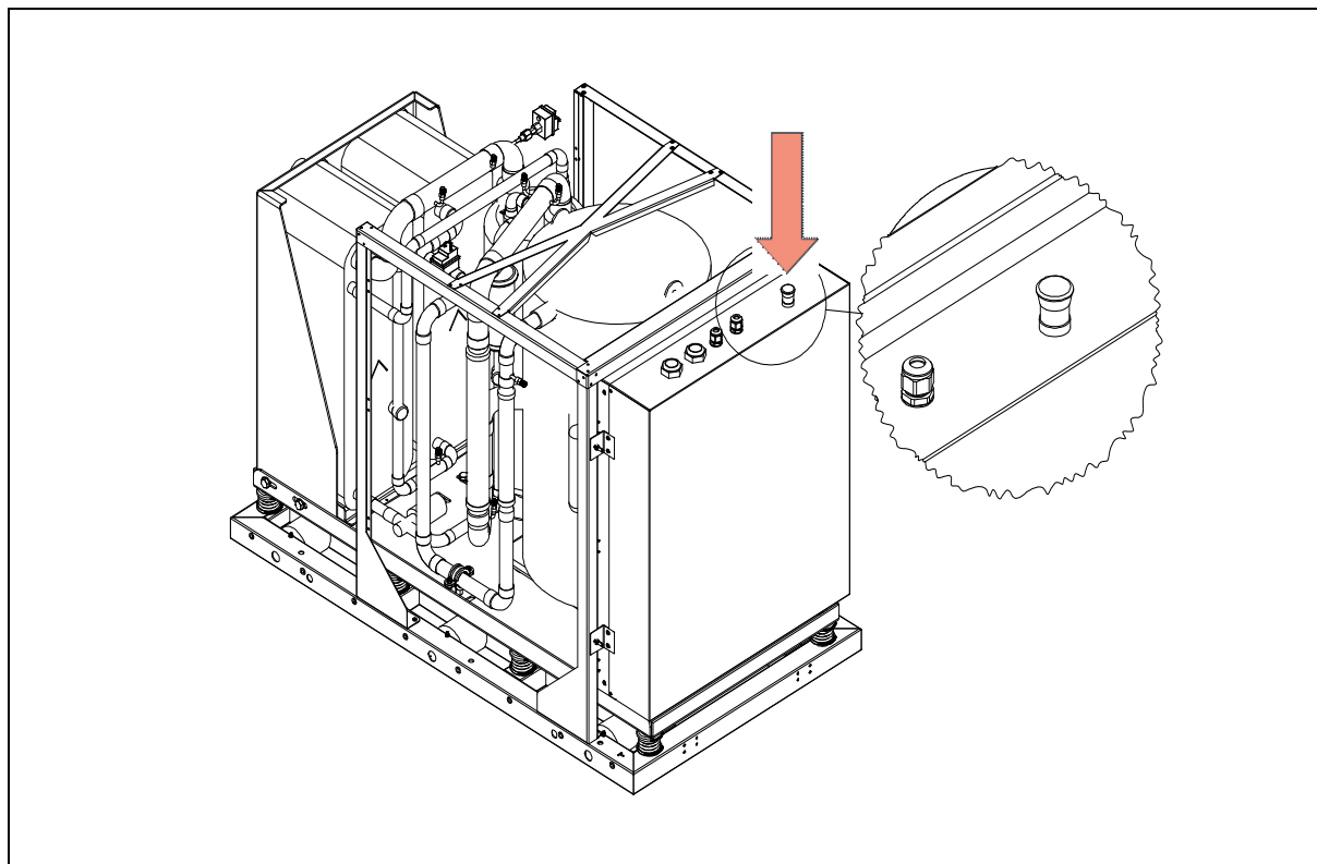
Rys. 19: Awaryjne zatrzymanie pompy ciepła przez wciśnięcie przycisku awaryjnego.
