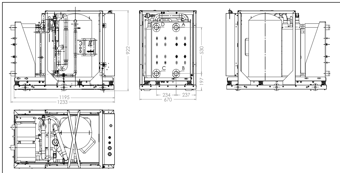
Rys. 3: Gabaryty pompy ciepła EUROS GEO PRO 3 w wersji MT.
