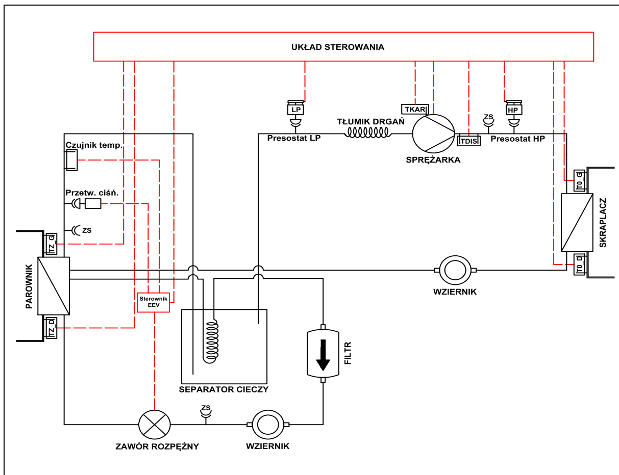
Rys. 2: Ogólny schemat układu chłodniczego i układu sterowania w pompach ciepła EUROS GEO PRO 3.
