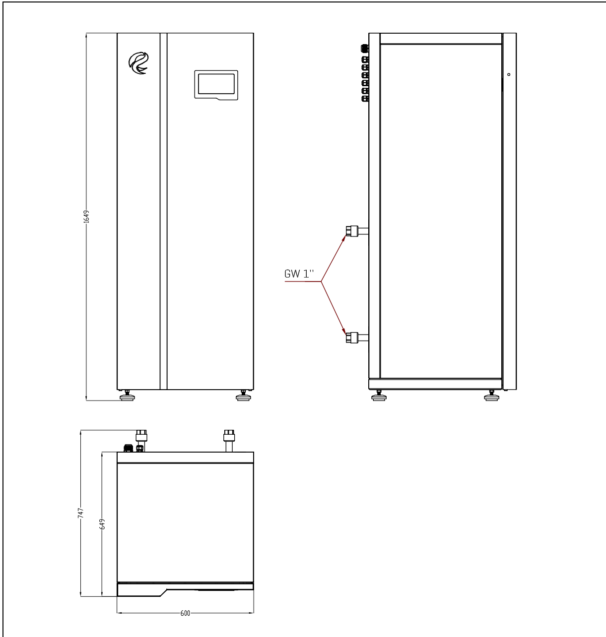
Rys. 6: Gabaryty jednostki wewnętrznej pompy ciepła EUROS GEO+.
