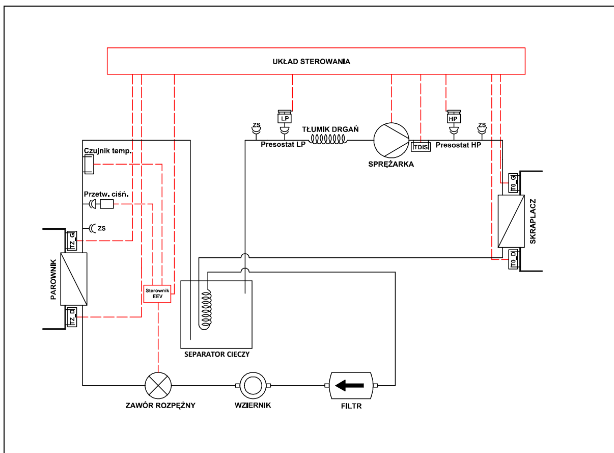
Rys. 4: Ogólny schemat układu chłodniczego i układu sterowania w pompach ciepła EUROS GEO+.
