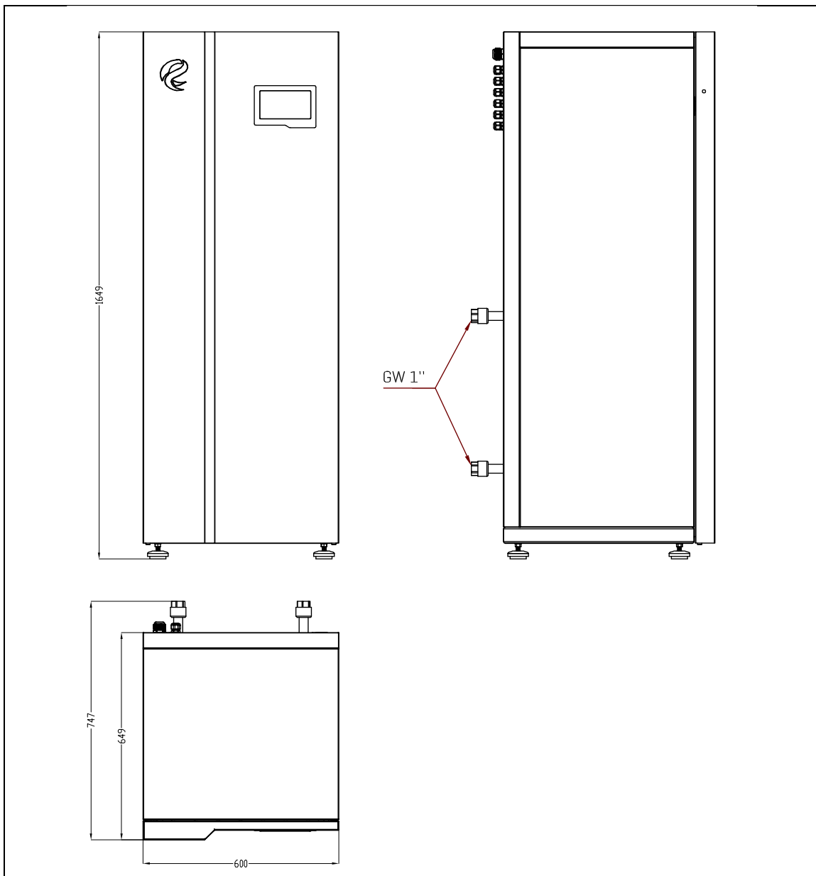
Rys. 6: Gabaryty jednostki wewnętrznej pompy ciepła EUROS GEO
