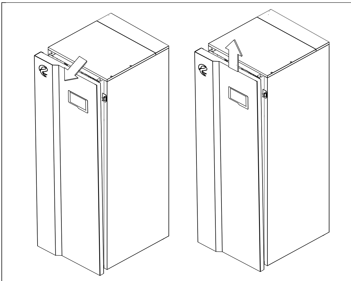
Rys. 10: Sposób otwierania frontowej osłony pompy ciepła EUROS GEO.
