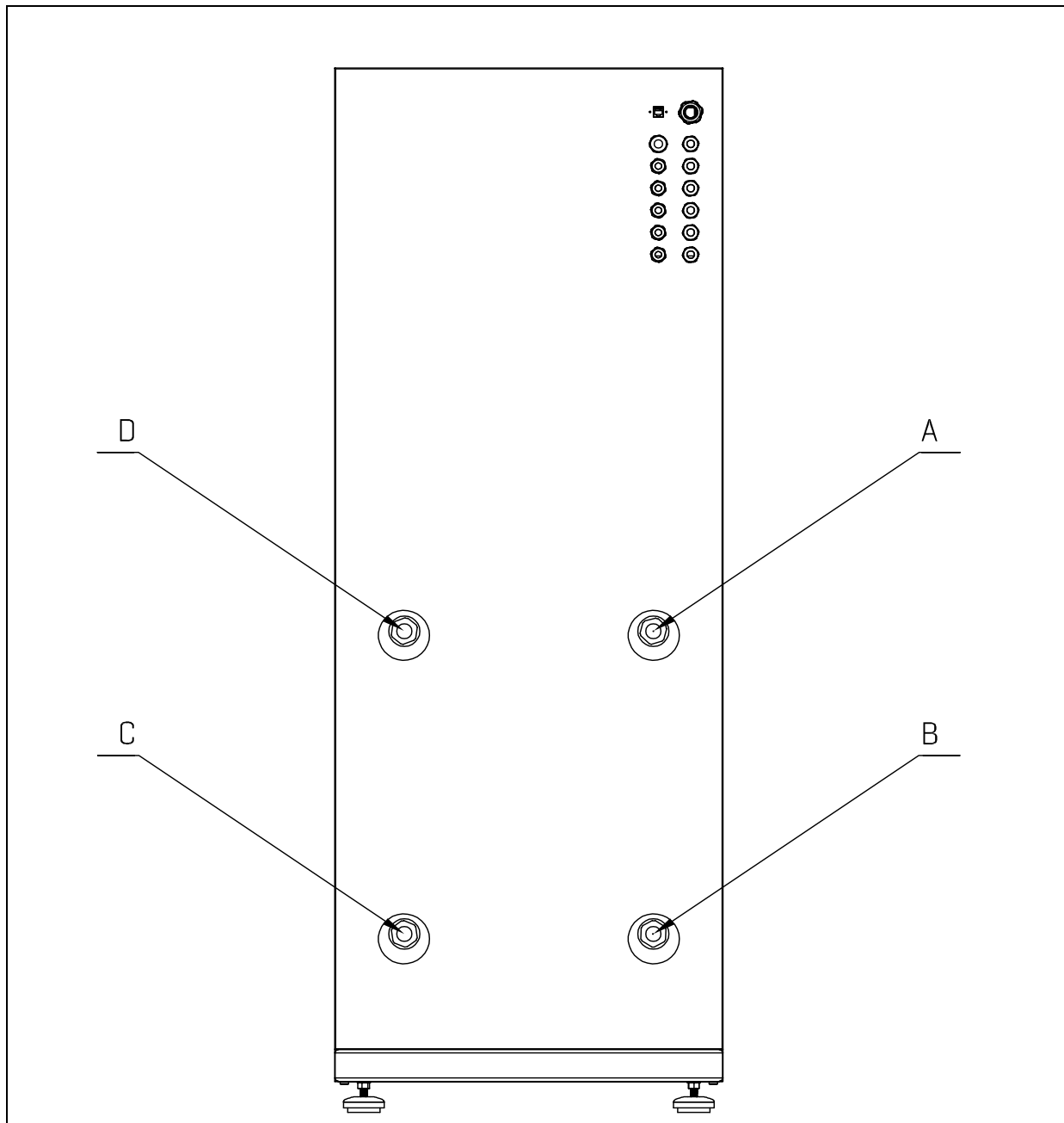
Rys. 9: Tylna strona obudowy pompy ciepła EUROS GEO.
