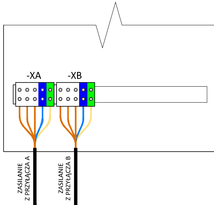
Rys. 29: Sposób przyłączenia zasilania do pompy ciepła EUROS CONTIBLOC MAXI dla wersji wykonania z dwoma przyłączami o mocach równych lub mniejszych niż 40 kW (tryb MPC)
