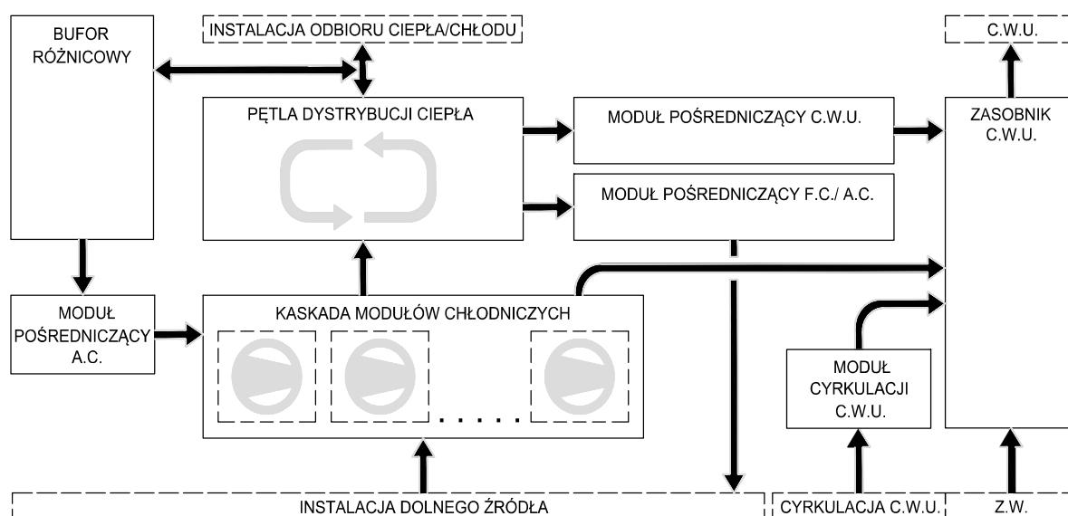
Rys. 2: Schemat blokowy pompy ciepła EUROS CONTIBLOC MAXI
