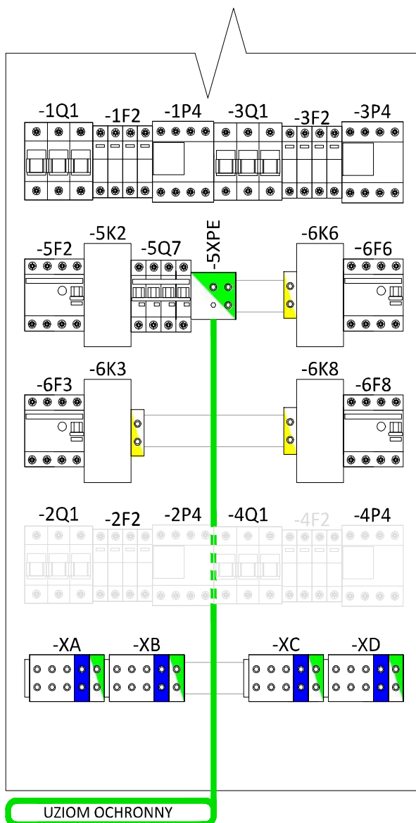
Rys. 34: Miejsce przyłączenia dodatkowego przewodu uziemiającego do pompy ciepła EUROS CONTIBLOC MAXI
