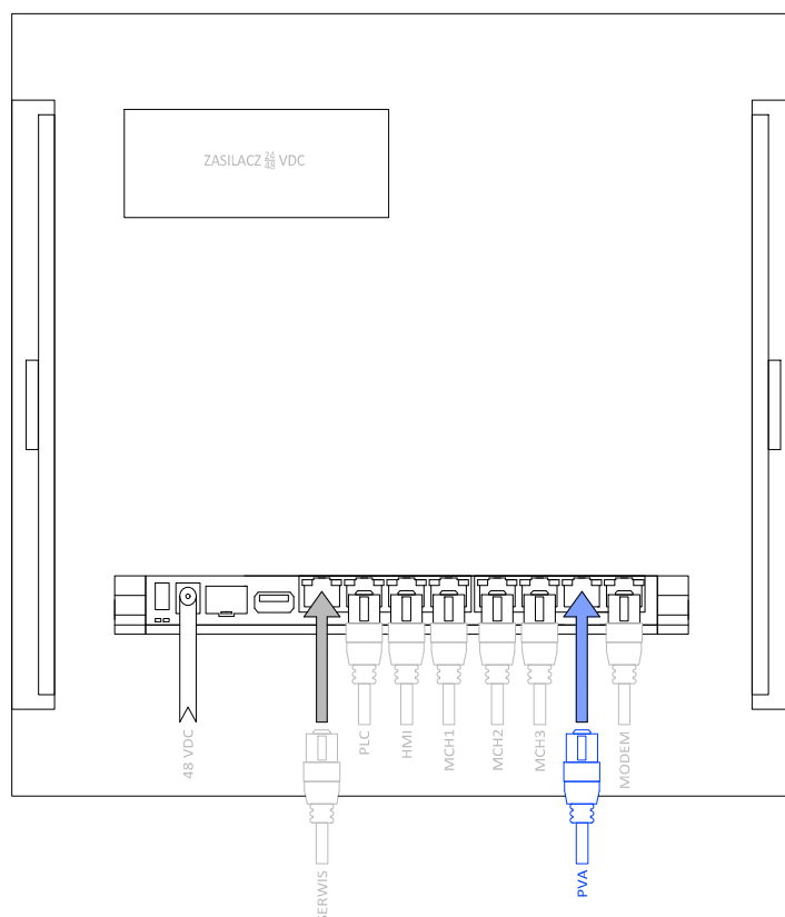
Rys. 36: Widok szafy komunikacyjnej i miejsce przyłączenia sygnałów komunikacyjnych z falowników PV dla wersji układu elektrycznego ECx12, ECx13
