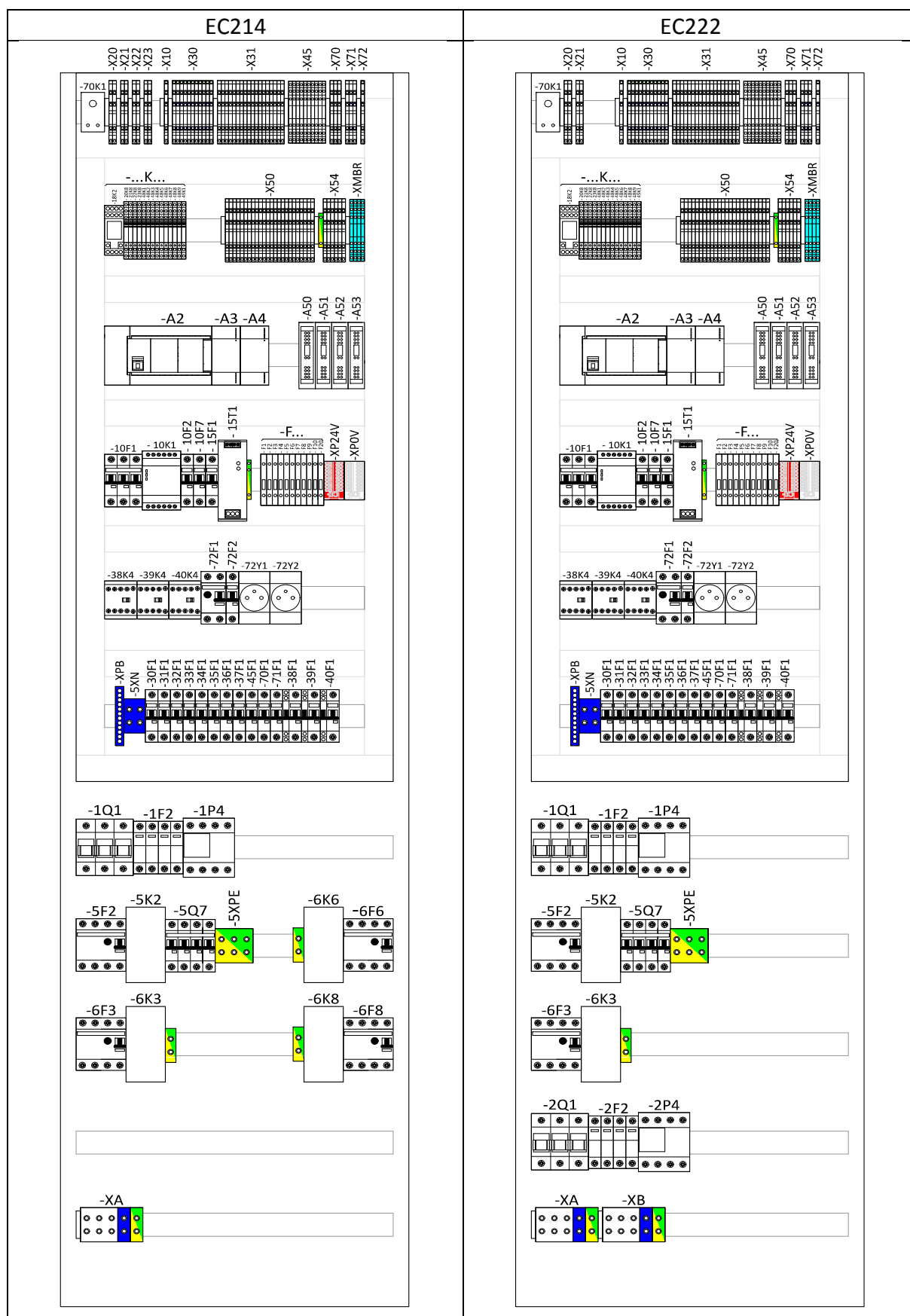
Rys.24: Widok aparatury w tablicy rozdzielczej w pompie ciepła EUROS CONTIBLOC MAXI (EC214, EC222)
