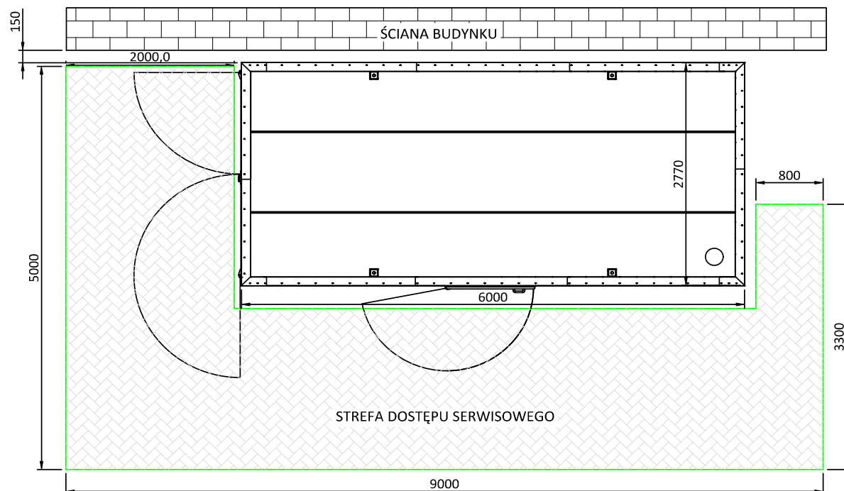
Rys. 12: Minimalne odstępy i strefy serwisowe
