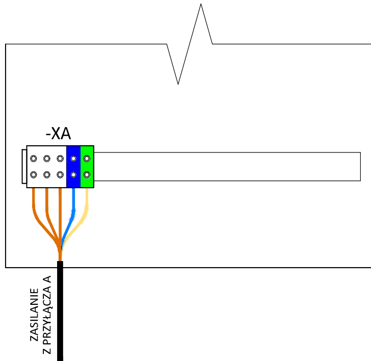
Rys. 28: Sposób przyłączenia zasilania do pompy ciepła EUROS CONTIBLOC MAXI dla wersji wykonania z jednym przyłączem o mocy równej lub mniejszej od 40 kW (tryb MPC)
