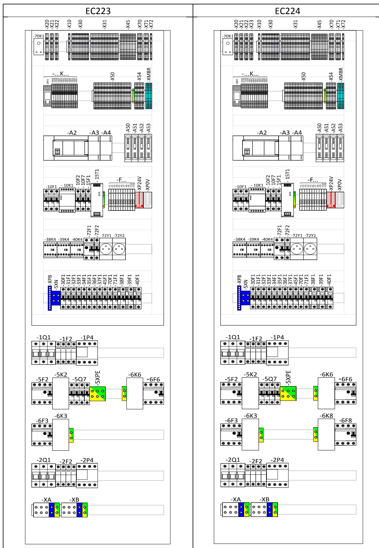
Rys.25: Widok aparatury w tablicy rozdzielczej w pompie ciepła EUROS CONTIBLOC MAXI (EC223, EC224)
