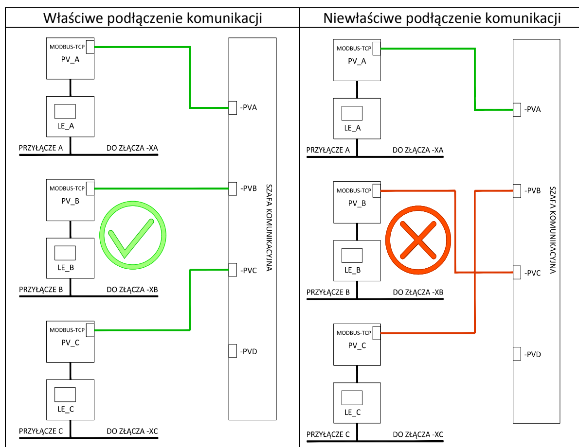
Rys. 35: Właściwe i niewłaściwe podłączenie komunikacji z falownikami PV
