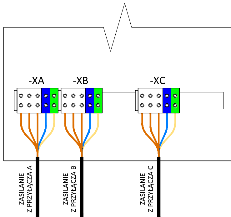
Rys. 30: Sposób przyłączenia zasilania do pompy ciepła EUROS CONTIBLOC MAXI dla wersji wykonania z trzema przyłączami o mocach równych lub mniejszych niż 40 kW (tryb MPC)
