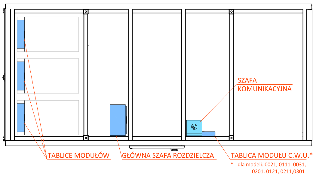
Rys. 20: Umieszczenie szaf i tablic elektrycznych w pompie ciepła EUROS CONTIBLOC MAXI
