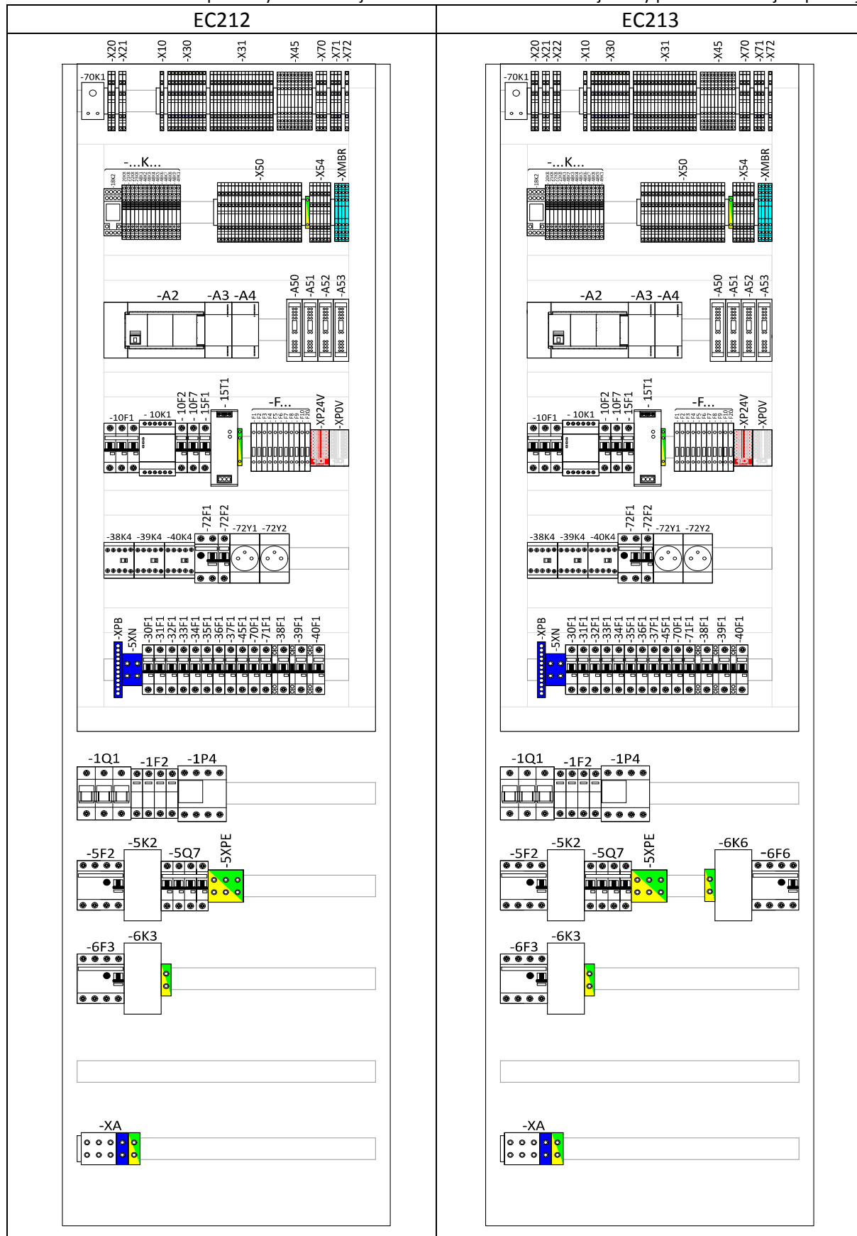
Rys.23: Widok aparatury w tablicy rozdzielczej w pompie ciepła EUROS CONTIBLOC MAXI (EC212, EC213)
