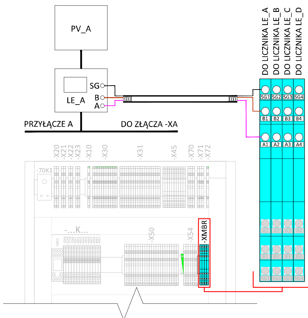
Rys. 38: Sposób podłączenia komunikacji poprzez MODBUS-RTU z licznikiem w obwodzie falownika PV
