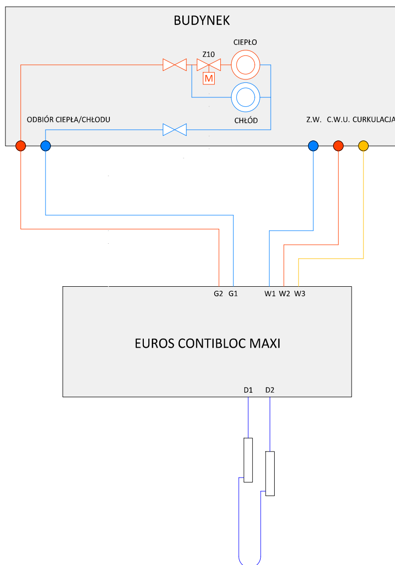
Rys. 15: Schemat aplikacyjny dla podłączenia hydraulicznego pompy ciepła EUROS CONTIBLOC MAXI – układ z dostarczaniem chłodu do wydzielonej części instalacji
