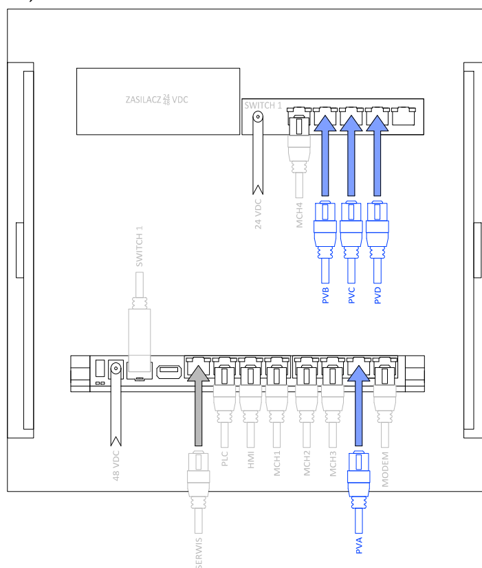
Rys. 37: Widok szafy komunikacyjnej i miejsce przyłączenia sygnałów komunikacyjnych MODBUS-TCP z falowników PV dla wersji układu elektrycznego ECx14, ECx22, ECx23, ECx24, ECx33, ECx34, ECx44
