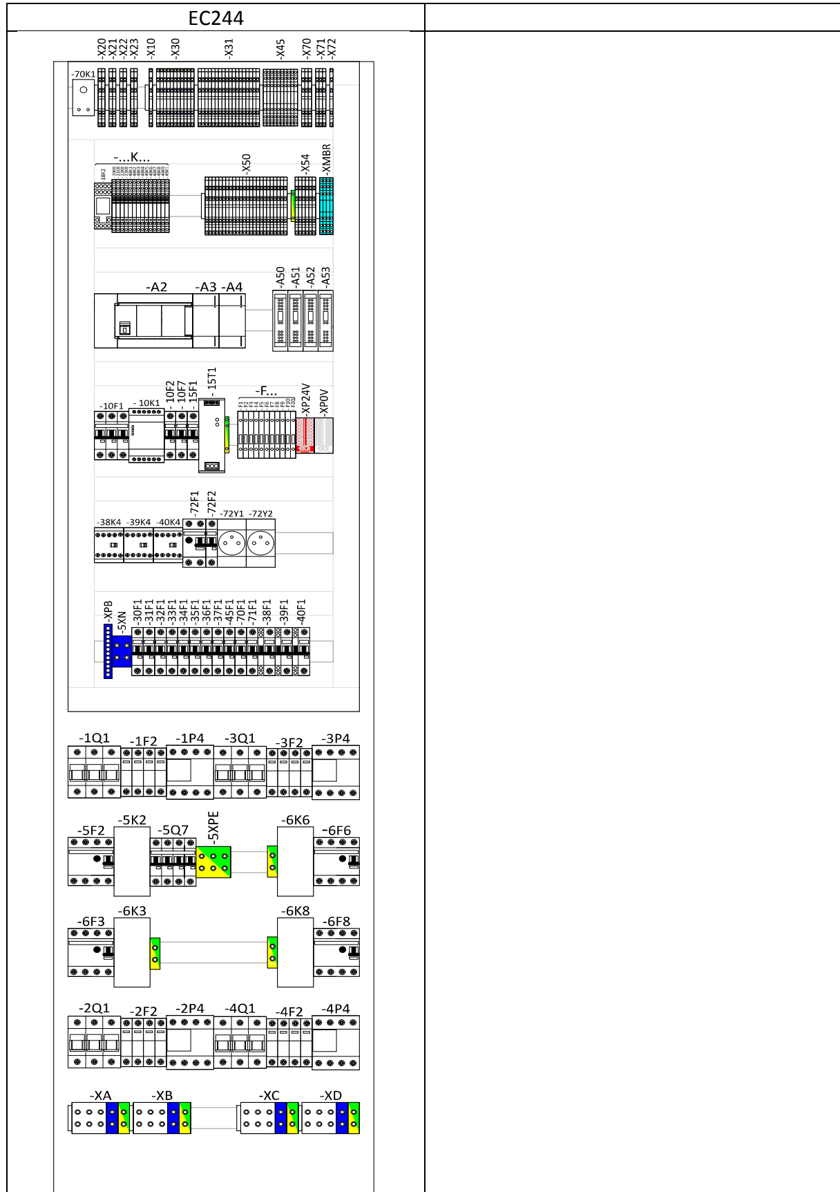
Rys.27: Widok aparatury w tablicy rozdzielczej w pompie ciepła EUROS CONTIBLOC MAXI (EC244)
