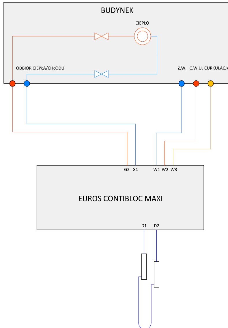
Rys. 14: Schemat aplikacyjny dla podłączenia hydraulicznego pompy ciepła EUROS CONTIBLOC MAXI – układ podstawowy
