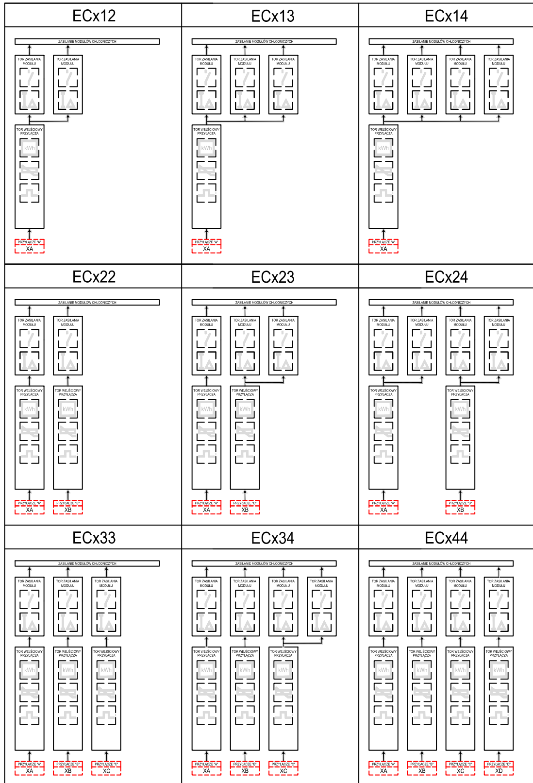
Rys. 21: Warianty sekcji mocy w pompie ciepła EUROS CONTIBLOC MAXI
