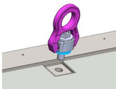
Rys. 6: Punkt mocujący w pompie ciepła EUROS CONTIBLOC MAXI
