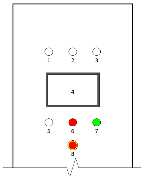
Rys. 22: Widok drzwi tablicy rozdzielczej w pompie ciepła EUROS CONTIBLOC MAXI
