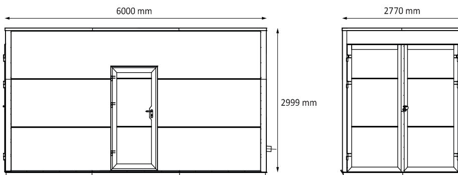
Rys. 4: Gabaryty pompy ciepła EUROS CONTIBLOC MAXI
