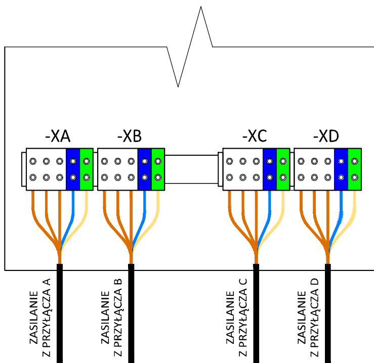
Rys. 31: Sposób przyłączenia zasilania do pompy ciepła EUROS CONTIBLOC MAXI dla wersji wykonania z czterema przyłączami o mocach równych lub mniejszych niż 40 kW (tryb MPC)
