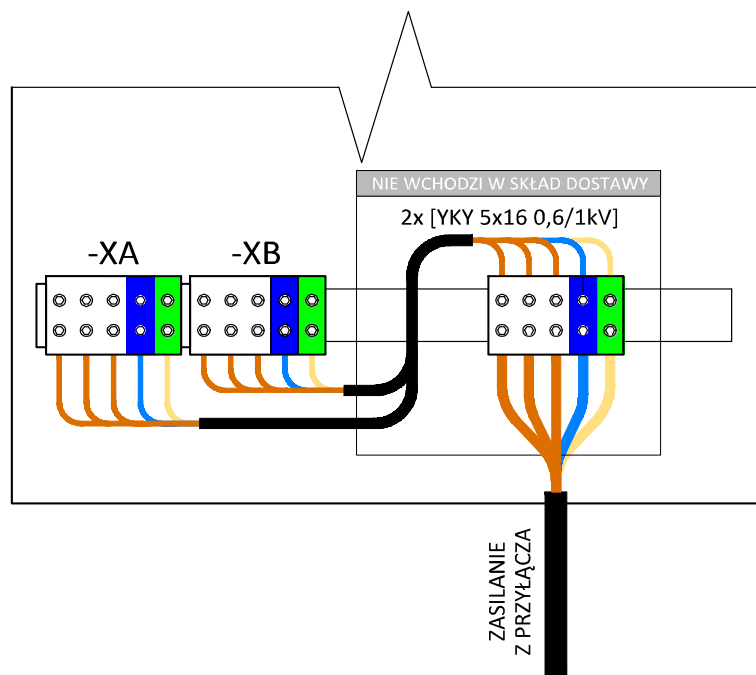
Rys. 32: Sposób przyłączenia zasilania do pompy ciepła EUROS CONTIBLOC MAXI z jednego przyłącza o znacznej mocy (tryb SPC) dla modeli 0021, 0110, 0030, 0111, 0031, 0201, 0121, R0211
