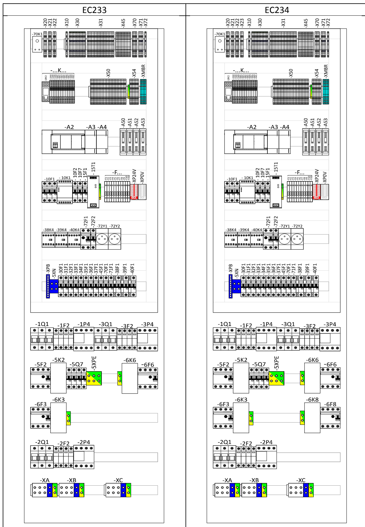
Rys.26: Widok aparatury w tablicy rozdzielczej w pompie ciepła EUROS CONTIBLOC MAXI (EC233, EC234)
