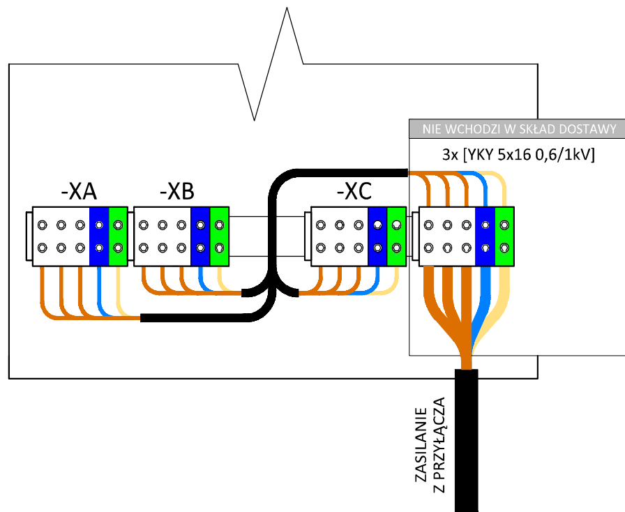
Rys. 33: Sposób przyłączenia zasilania do pompy ciepła EUROS CONTIBLOC MAXI z jednego przyłącza o znacznej mocy (tryb SPC) dla modeli 0211, 0300, 0301
