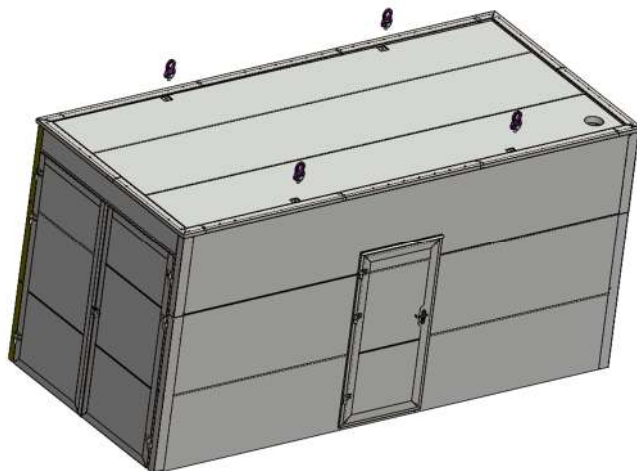
Rys. 5: Rozmieszczenie transportowych punktów mocujących w pompie ciepła EUROS CONTIBLOC MAXI
