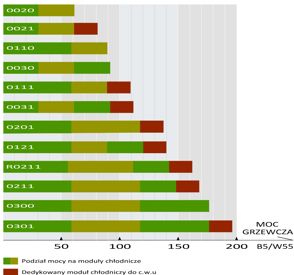
Rys. 3: Zestawienie mocy grzewczej różnych modeli pomp ciepła EUROS CONTIBLOC MAXI
