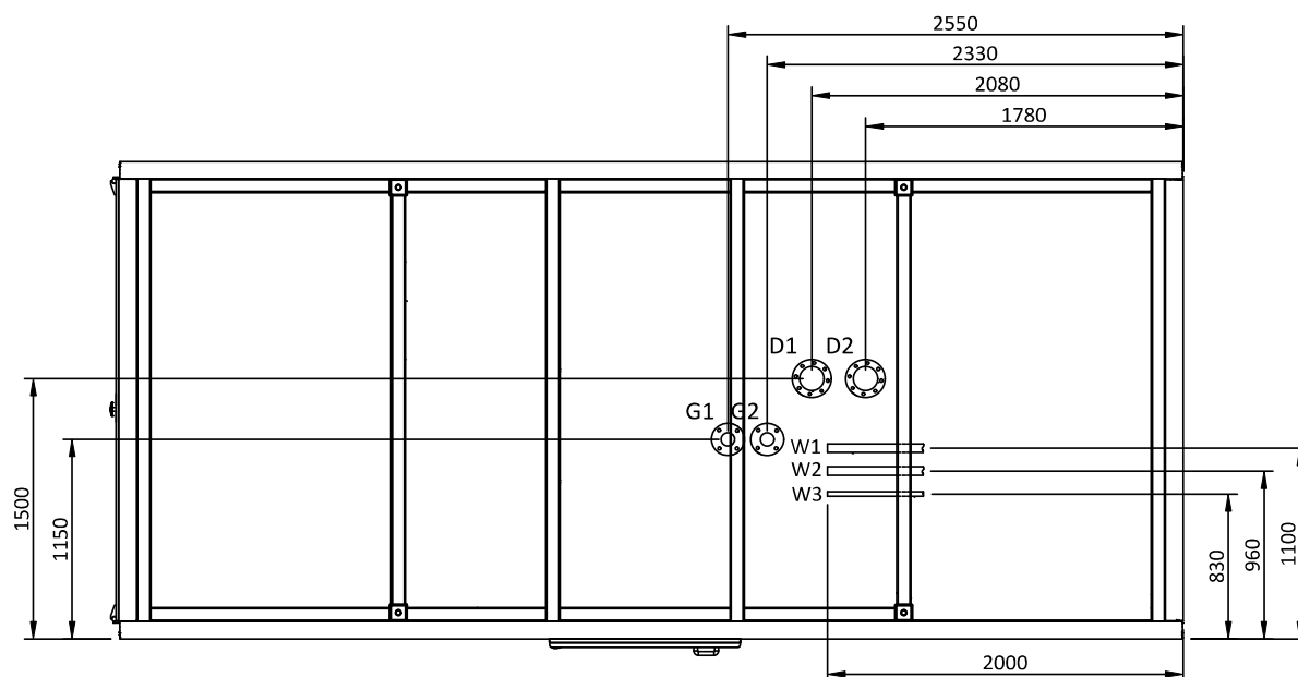
Rys. 13: Umieszczenie przyłączy hydraulicznych w odniesieniu do podstawy pompy ciepła EUROS CONTIBLOC MAXI
