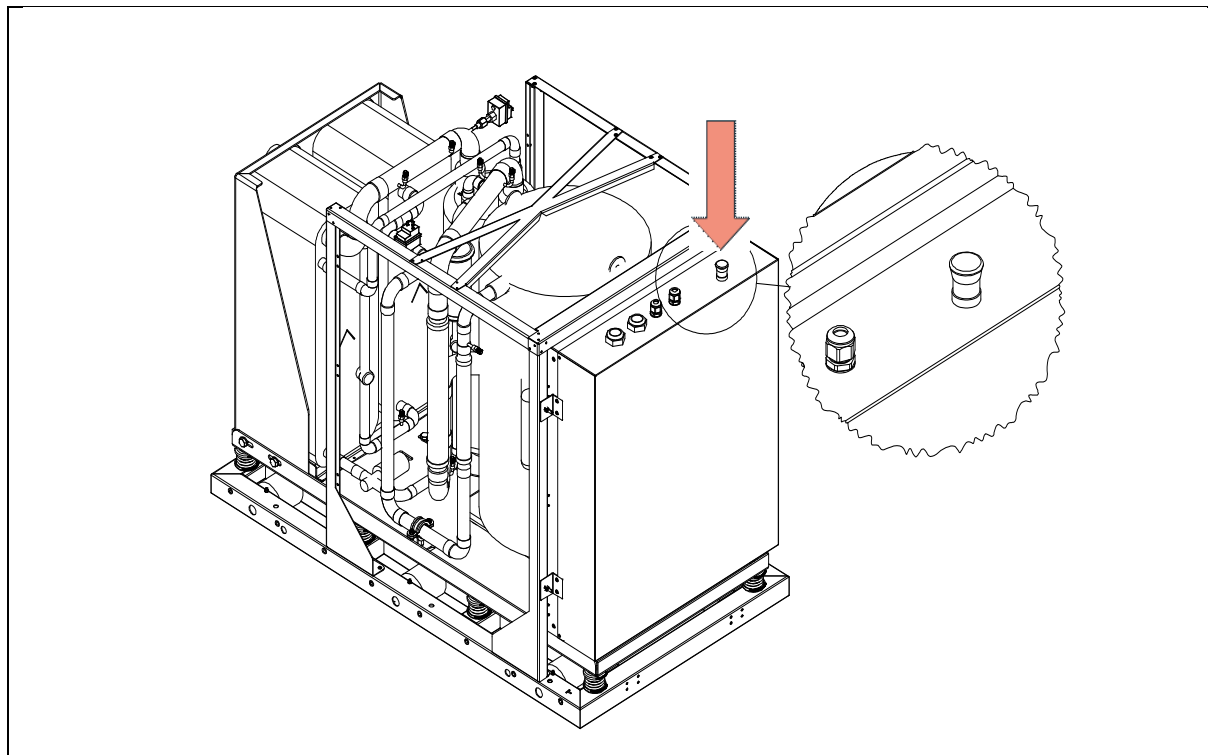
Rys. 40: Umieszczenie przycisku awaryjnego zatrzymania modułu chłodniczego
