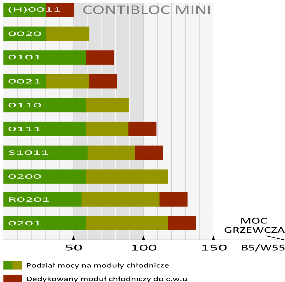
Rys. 3: Zestawienie mocy grzewczej różnych modeli pomp ciepła EUROS CONTIBLOC MINI.
