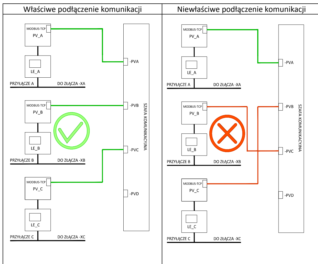
Rys. 39: Właściwe i niewłaściwe podłączenie komunikacji z falownikami PV.
