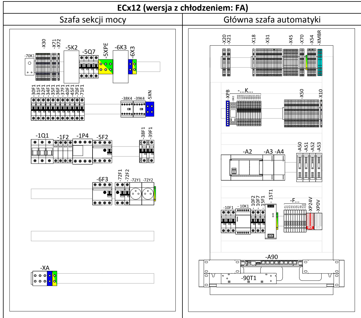
Rys. 23: Widok aparatury w tablicach rozdzielczych w pompie ciepła EUROS CONTIBLOC MINI (ECx12) (wersja z chłodzeniem: FA).
