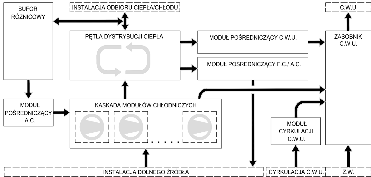
Rys. 2: Schemat blokowy pompy ciepła EUROS CONTIBLOC MINI.
