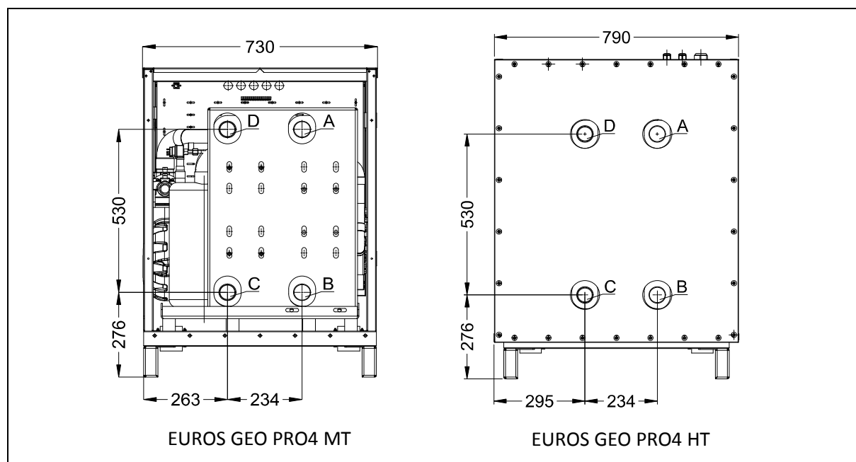
Rys. 13: Przyłącza hydrauliczne pompy ciepła EUROS GEO PRO4.
