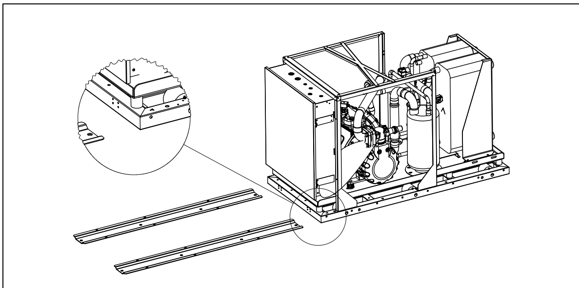
Rys. 9: Nakierowanie pompy ciepła na szyny montażowe.
