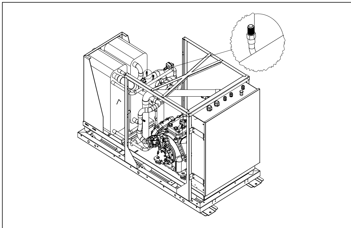
Rys. 20: Usytuowanie zaworów serwisowych w pompie ciepła EUROS GEO PRO4.
