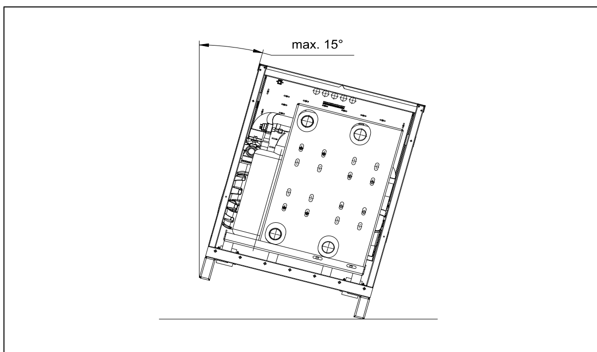
Rys. 5: Maksymalny przechył pompy ciepła EUROS GEO PRO4 w czasie transportu.
