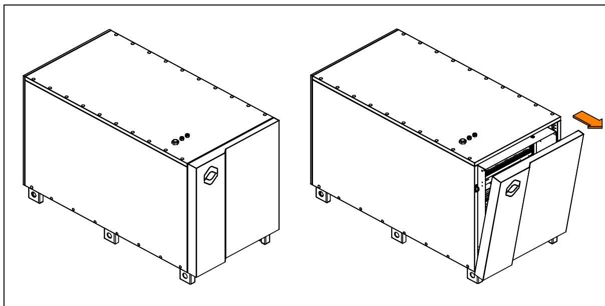
Rys. 18: Sposób zdejmowania panelu przedniego obudowy pompy ciepła EUROS GEO PRO4 w wersji HT.
