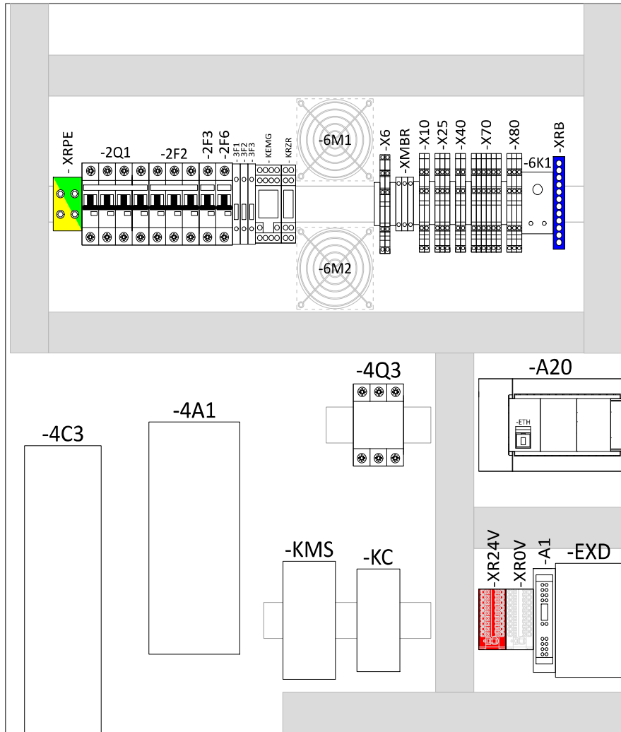
Rys. 15: Tablica elektryczna pompy ciepła EUROS GEO PRO4 w wersji ETO1.
