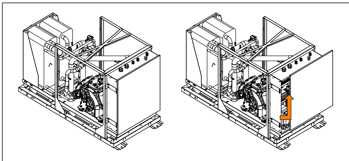
Rys. 17: Sposób zdejmowania panelu tablicy elektrycznej pompy ciepła EUROS GEO PRO4 w wersji MT.
