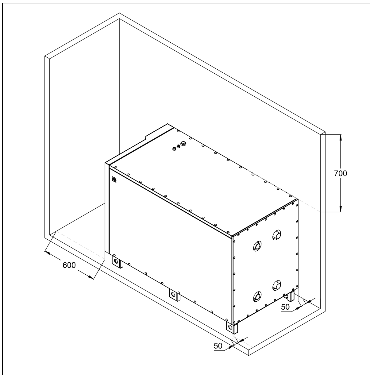
Rys. 7: Ograniczenia dotyczące miejsca ustawienia pompy ciepła EUROS GEO PRO4 HT z wyjątkiem pracy w kaskadzie.
