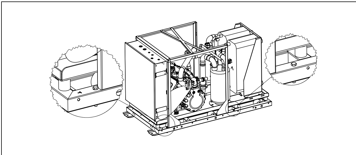
Rys. 12: Wkręcenie śrub blokujących w ramę modułu pompy ciepła.
