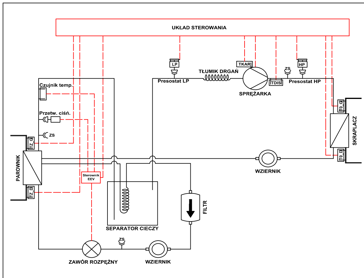
Rys. 2: Ogólny schemat układu chłodniczego i układu sterowania w pompach ciepła EUROS GEO PRO4.
