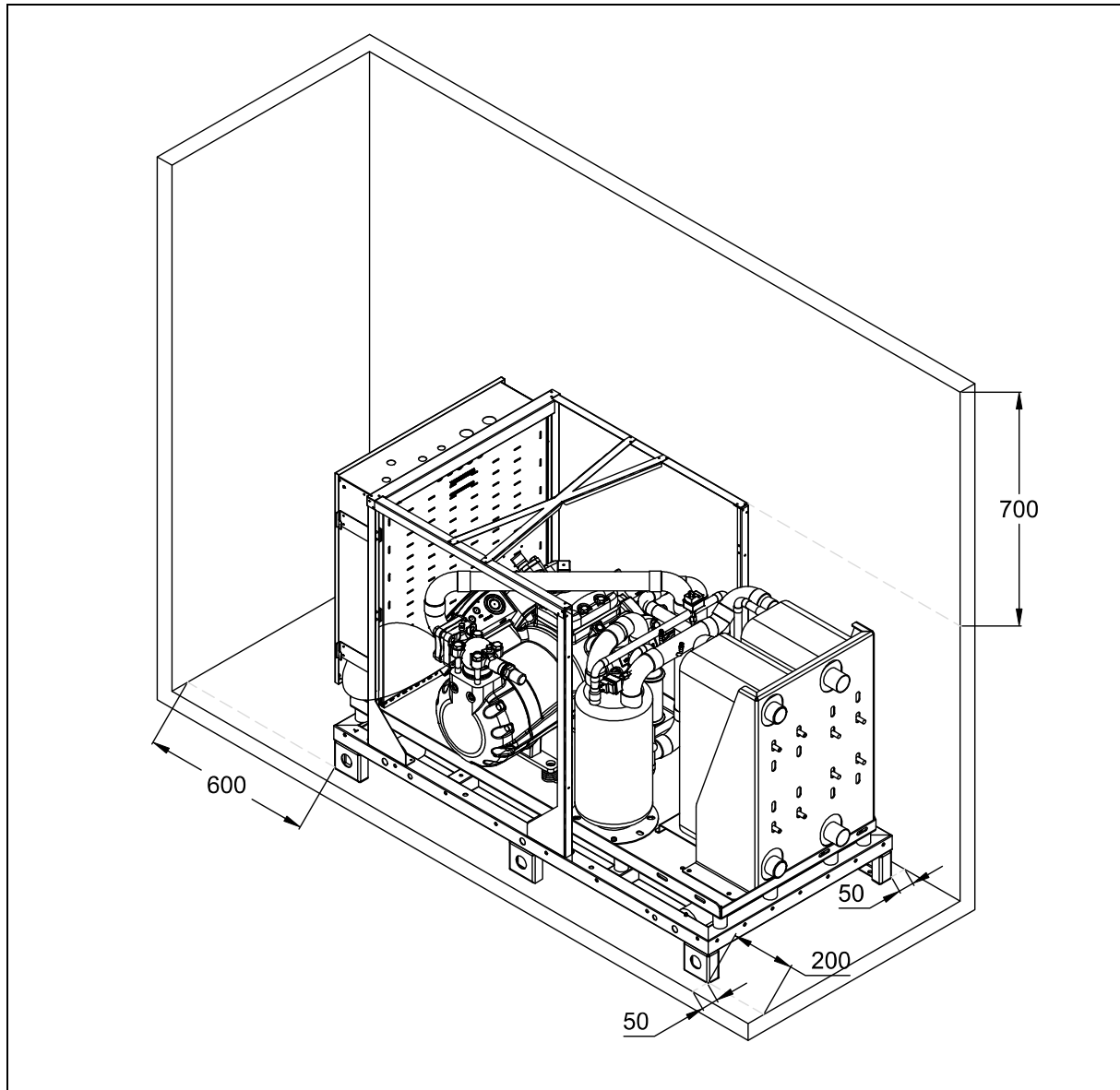
Rys. 6: Ograniczenia dotyczące miejsca ustawienia pompy ciepła EUROS GEO PRO4 MT z wyjątkiem pracy w kaskadzie.
