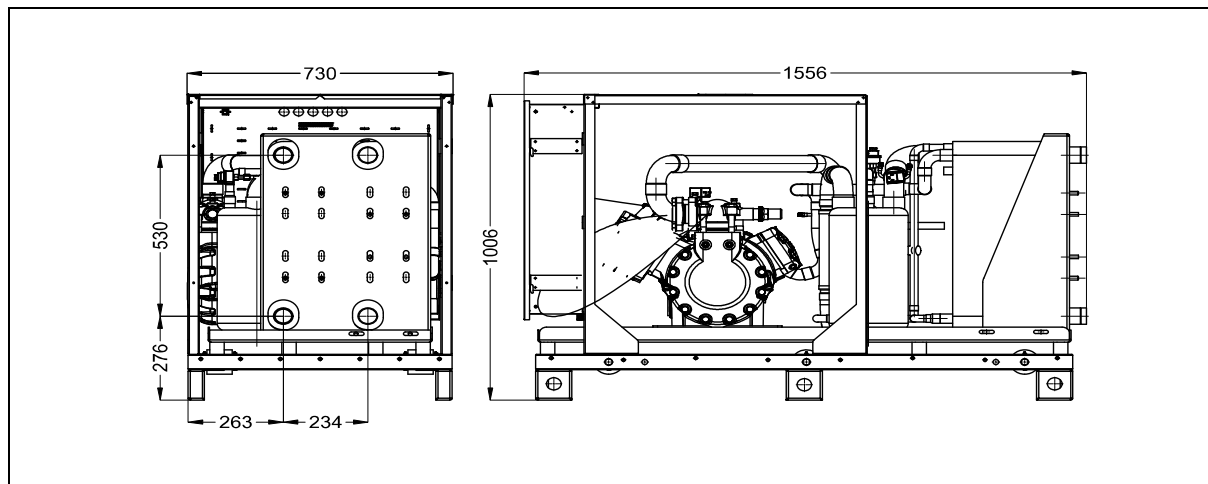
Rys. 3: Gabaryty pompy ciepła EUROS GEO PRO4 w wersji MT.
