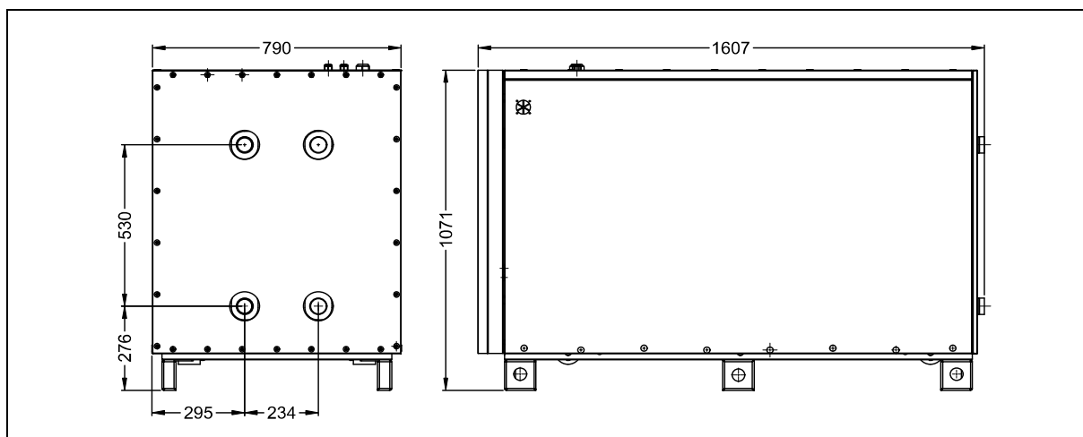
Rys. 4: Gabaryty pompy ciepła EUROS GEO PRO4 w wersji HT.
