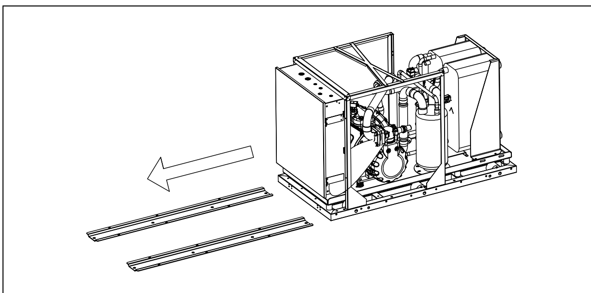
Rys. 10: Wsuniecie pompy ciepła na szyny montażowe.
