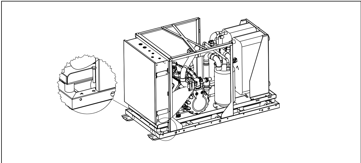
Rys. 11: Wsuniecie śrub blokujących w otwory umieszczone w ramie.
